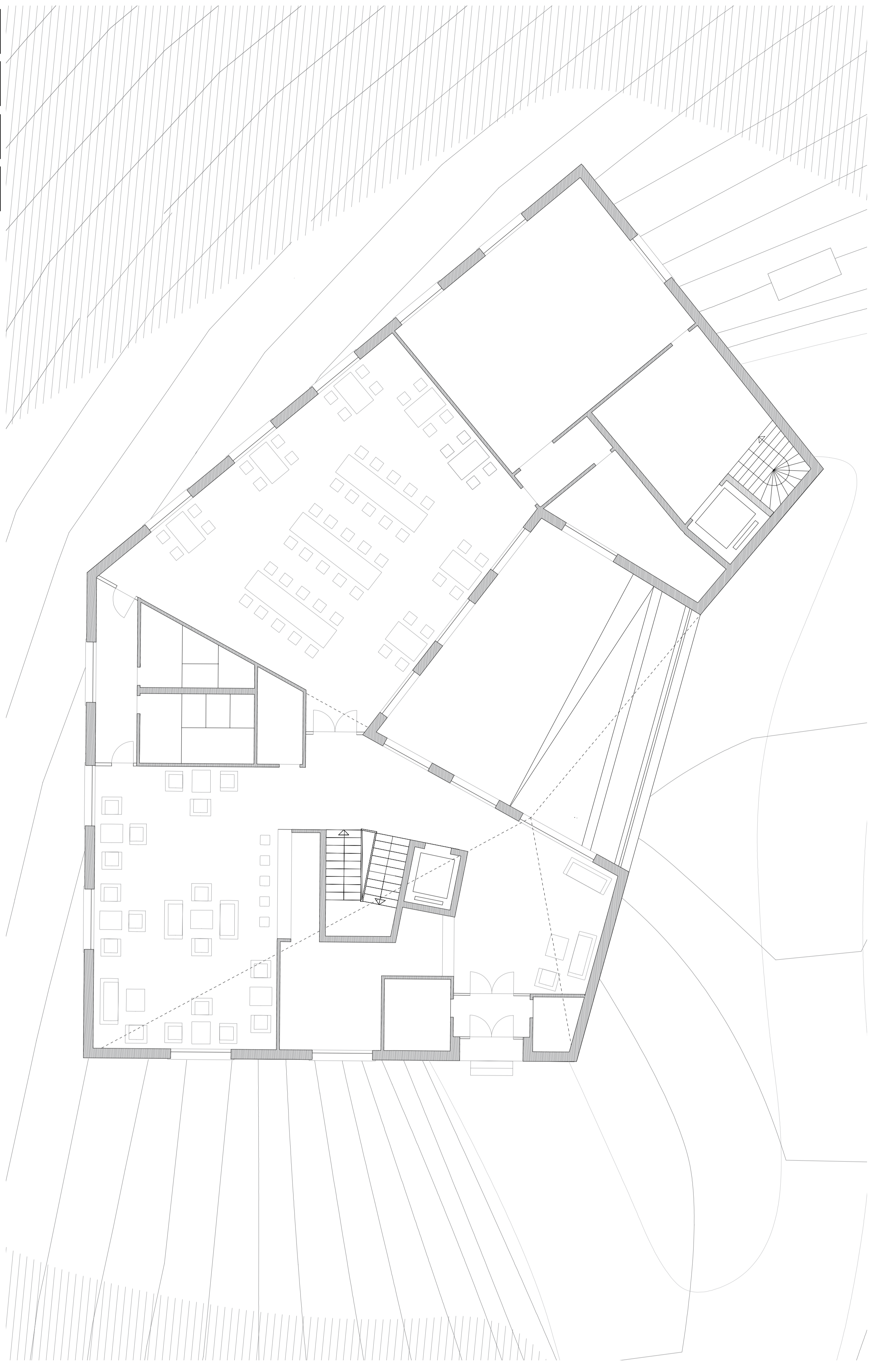
grundriss 4 og 1_100 eingang_rezeption_lobby_restaurant
