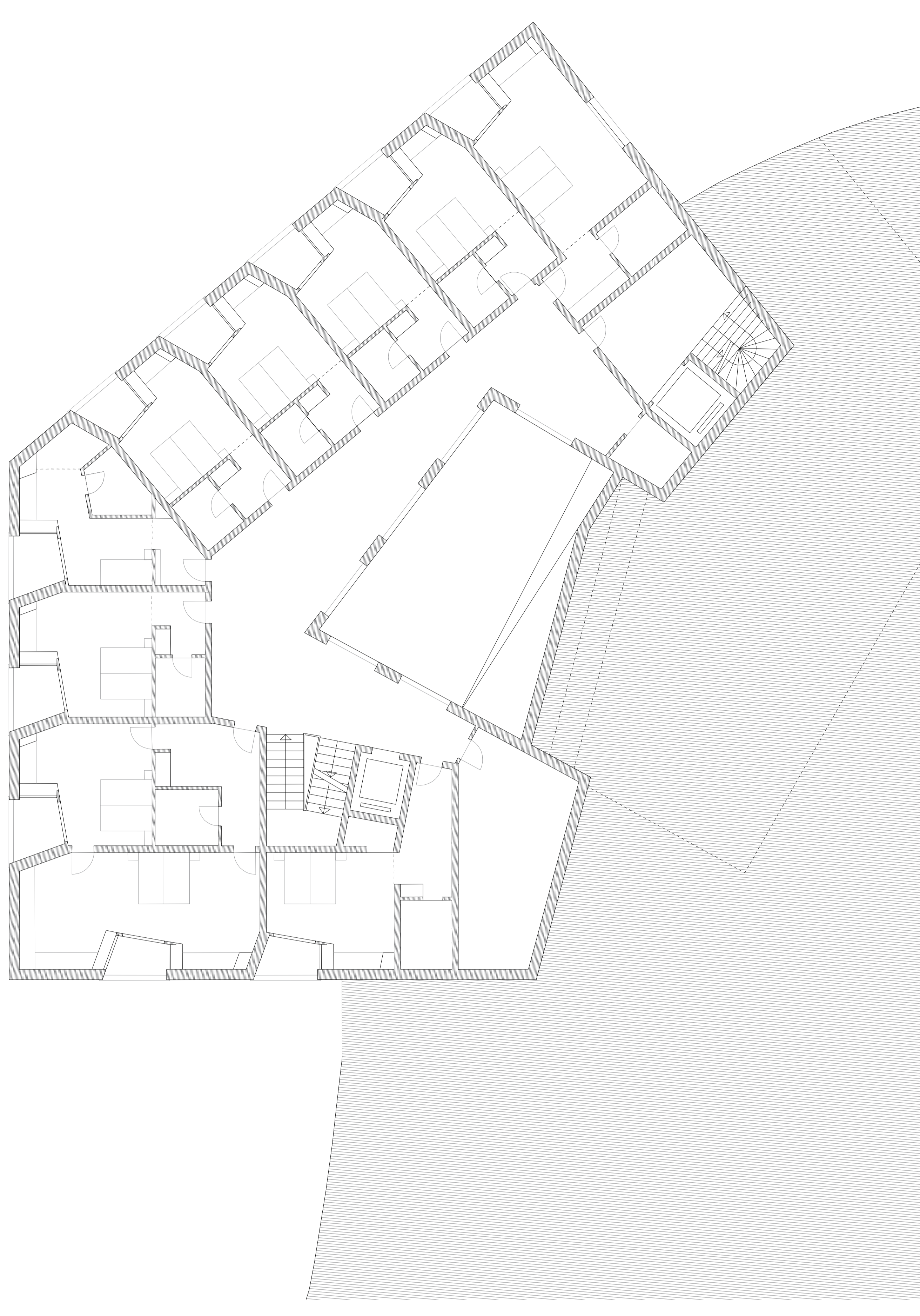
grundriss regelgeschoss 1_100 zimmer_etagenlager
