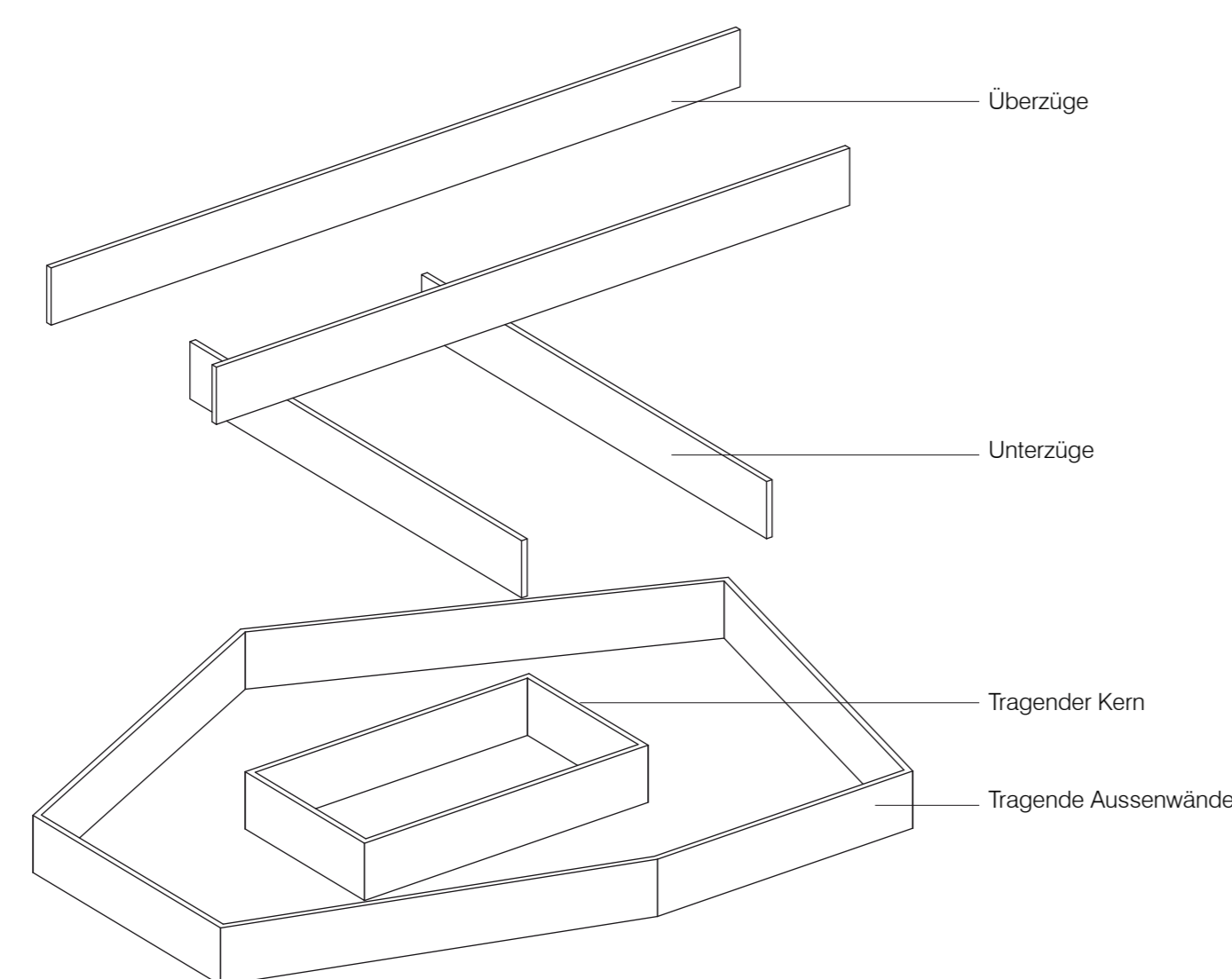
Tragprinzip
