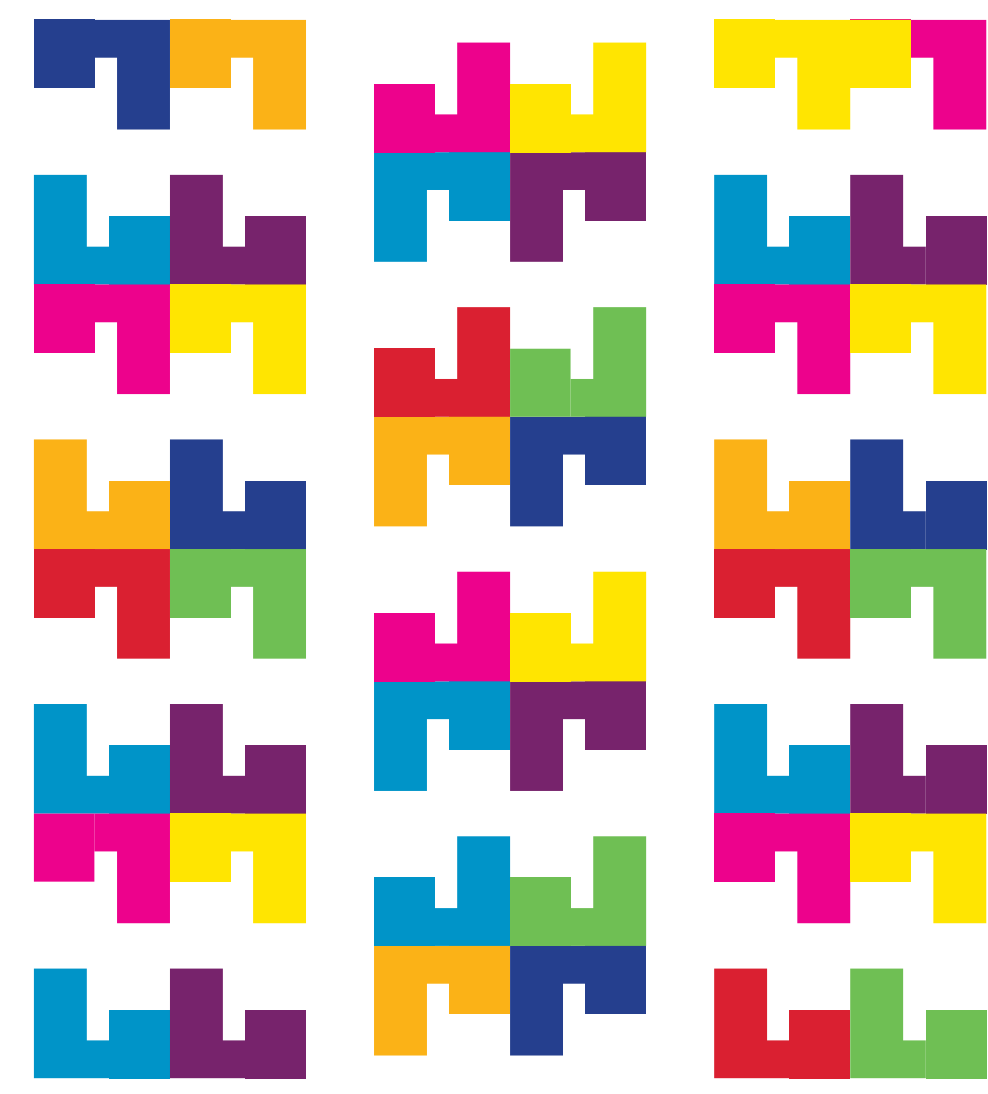
Kombinatorik
