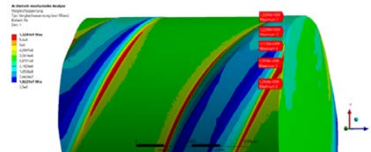
Abbildung 3: Vergleichsspannungen nach von Mises, verkürztes Rippenmodell
