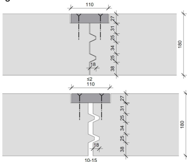
Bild 4 Darstellung von zwei beispielhaften Elementstößen der Brettschichtholzdecke
