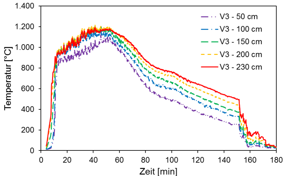
Bild 12 Temperatur-Zeit-Verläufe V3 im Brandraum in verschiedenen Höhen (Mittelwert)
