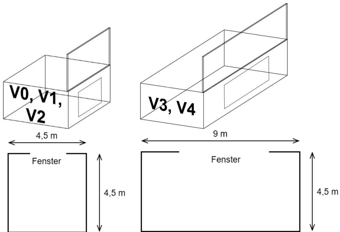
Bild 3 Grundrisse der fünf Realbrandversuche
