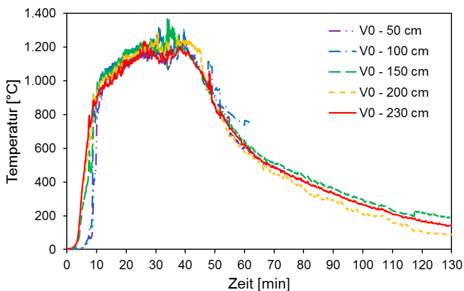
Bild 6 Temperatur-Zeit-Verläufe V0 im Brandraum in verschiedenen Höhen (Mittelwert)
