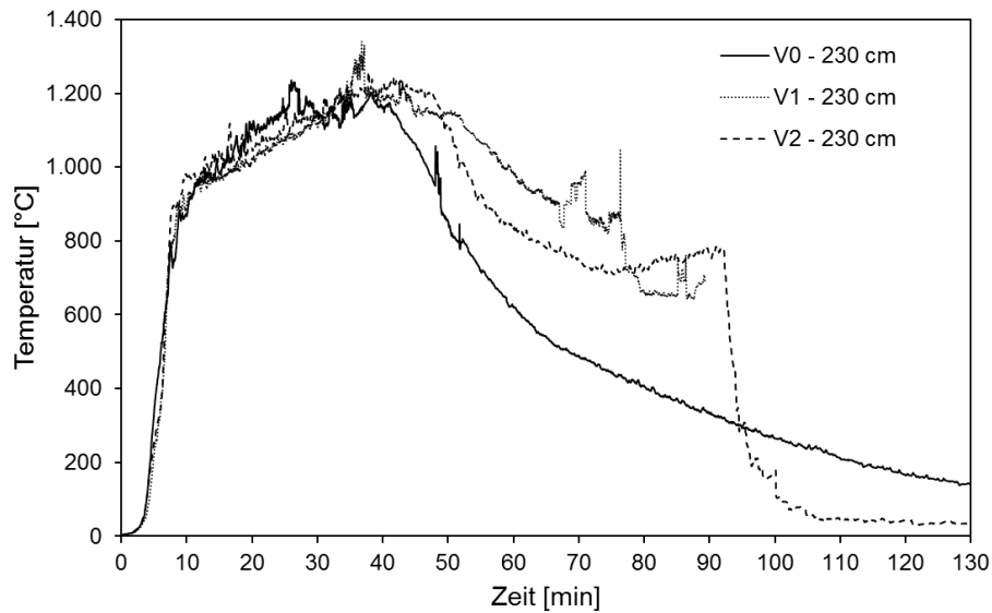
Bild 15 Vergleich Temperatur-Zeit-Verläufe V0, V1, V2 im Brandraum in 230 cm Höhe (Mittelwert)
