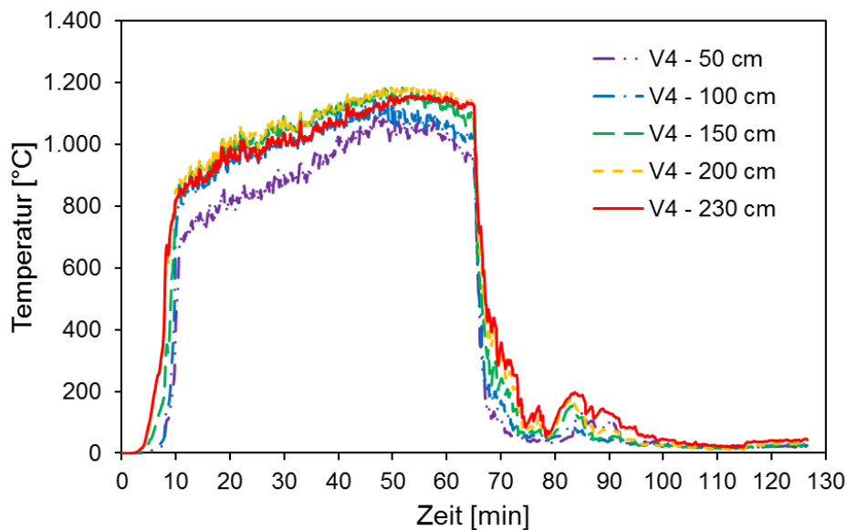
Bild 14 Temperatur-Zeit-Verläufe V4 im Brandraum in verschiedenen Höhen (Mittelwert)
