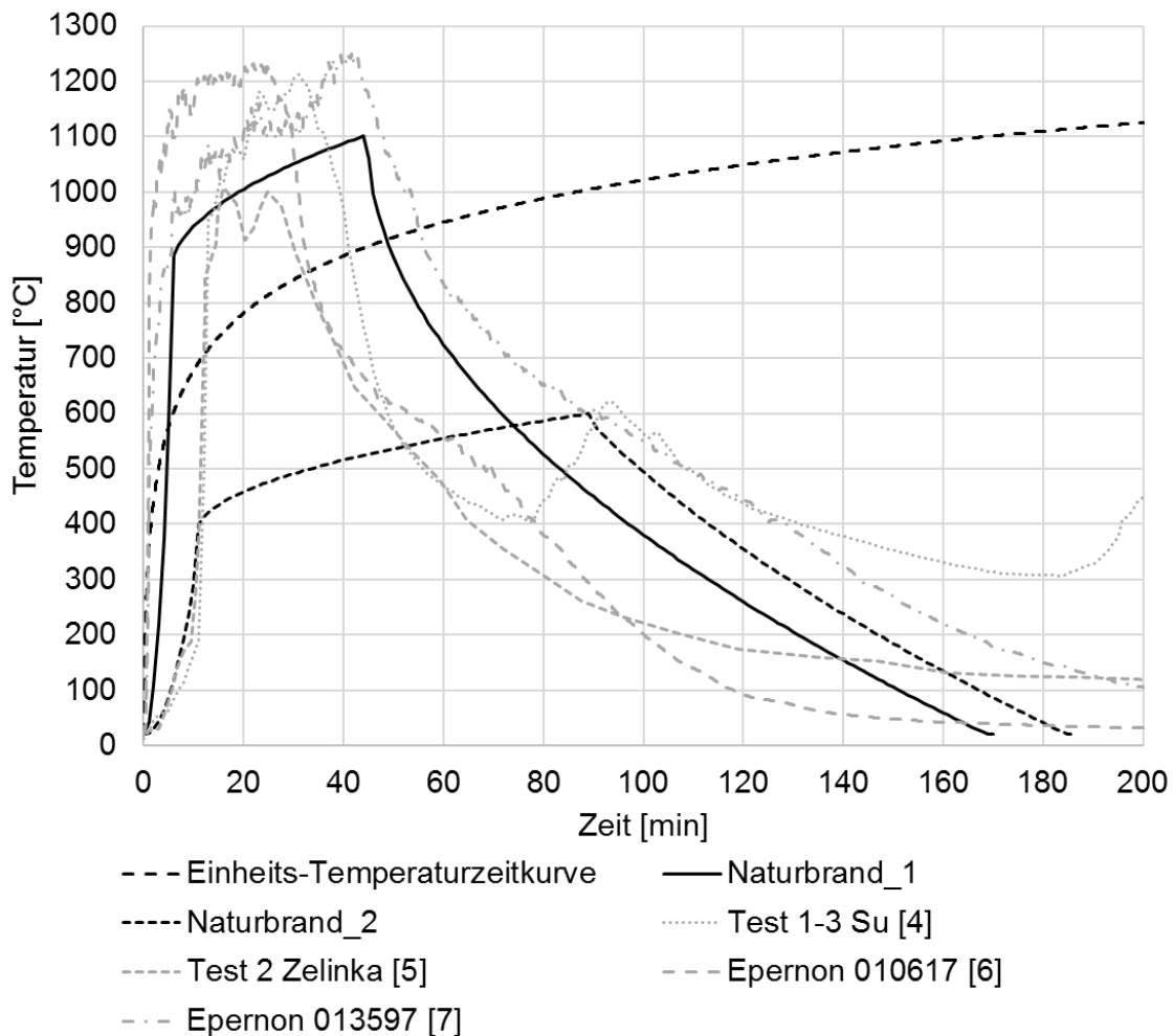
Bild 1: Die beiden gewählten repräsentativen Naturbrandkurven im Vergleich zur ETK sowie zu experimentellen Brandkurven
