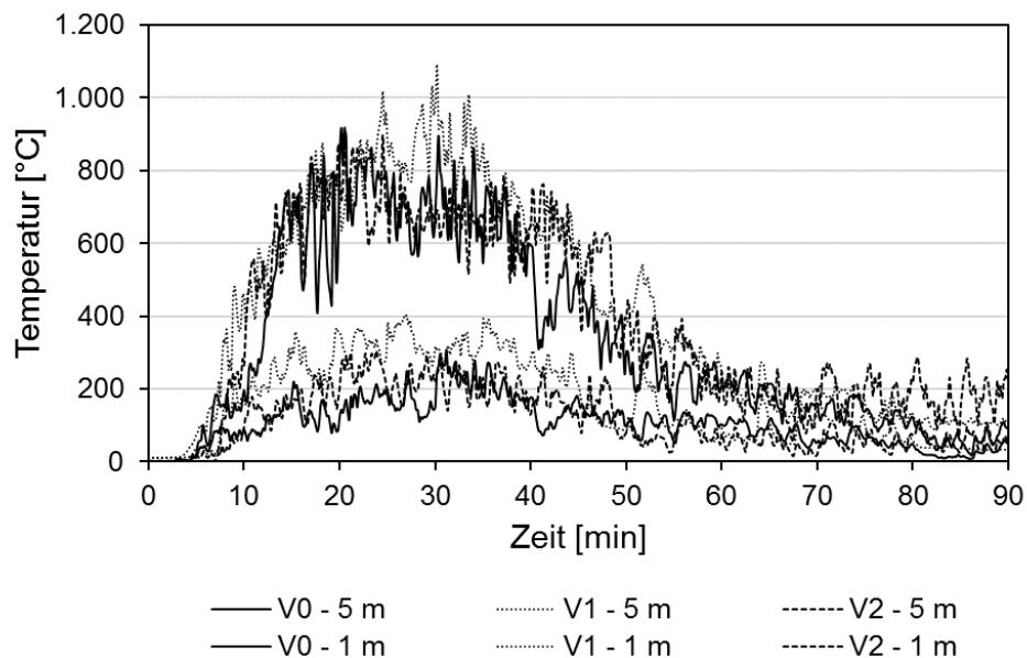
Bild 16 Vergleich der Temperatur-Zeit-Verläufe in der Mitte des Fassadenschildes in den Höhe 1 m und 5 m über die Brandraumöffnung für die Versuche V0, V1, V2
