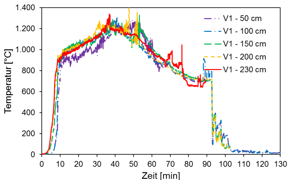
Bild 8 Temperatur-Zeit-Verläufe V1 im Brandraum in verschiedenen Höhen (Mittelwert)
