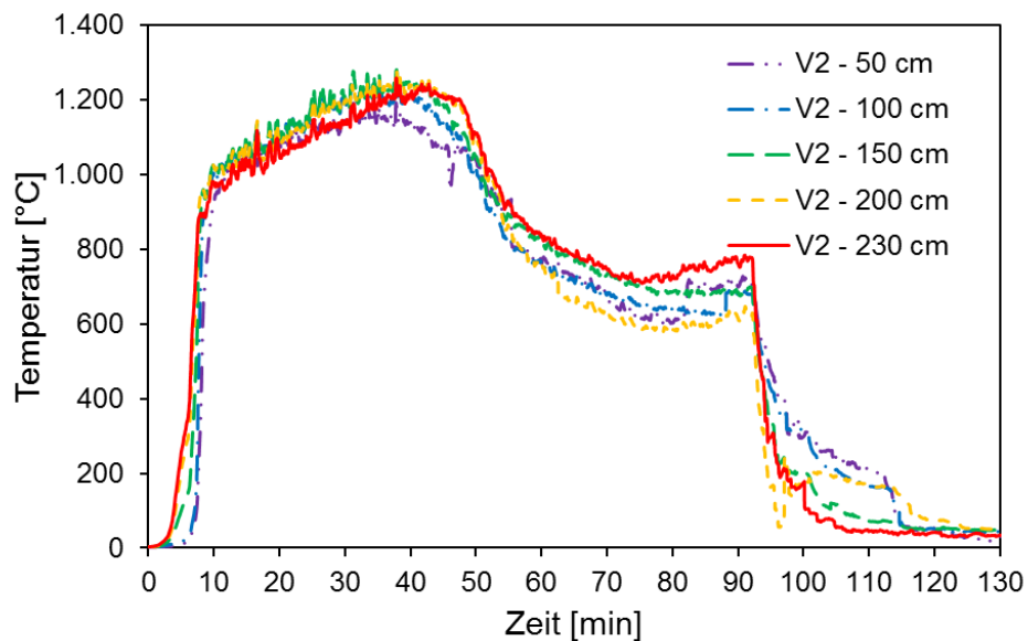
Bild 10 Temperatur-Zeit-Verläufe V2 im Brandraum in verschiedenen Höhen (Mittelwert)
