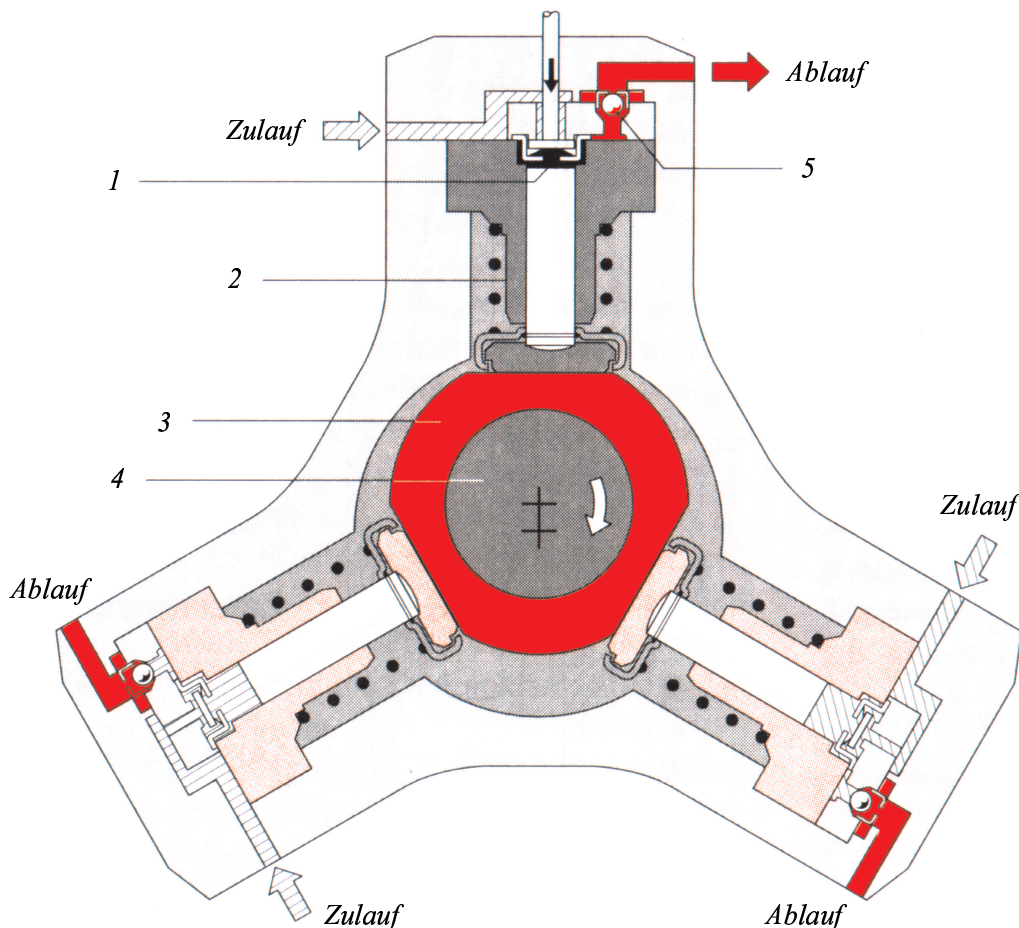
Abbildung 2.11: Common-Rail Hochdruckpumpe
