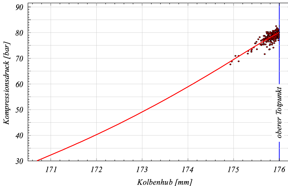
Abbildung 6.5: Erreichter Kompressionsdruck bei unterschiedlichen Kolbenhuben (300 Einzelversuche) mit konstantem Antriebsdruck
