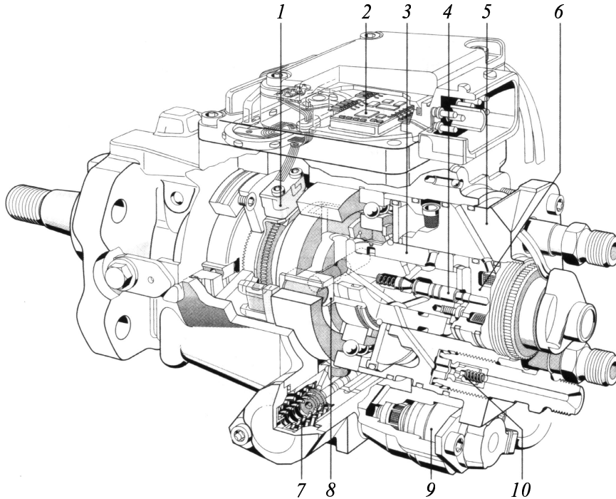
Abbildung 2.3: Radialkolben-Verteilereinspritzpumpe
