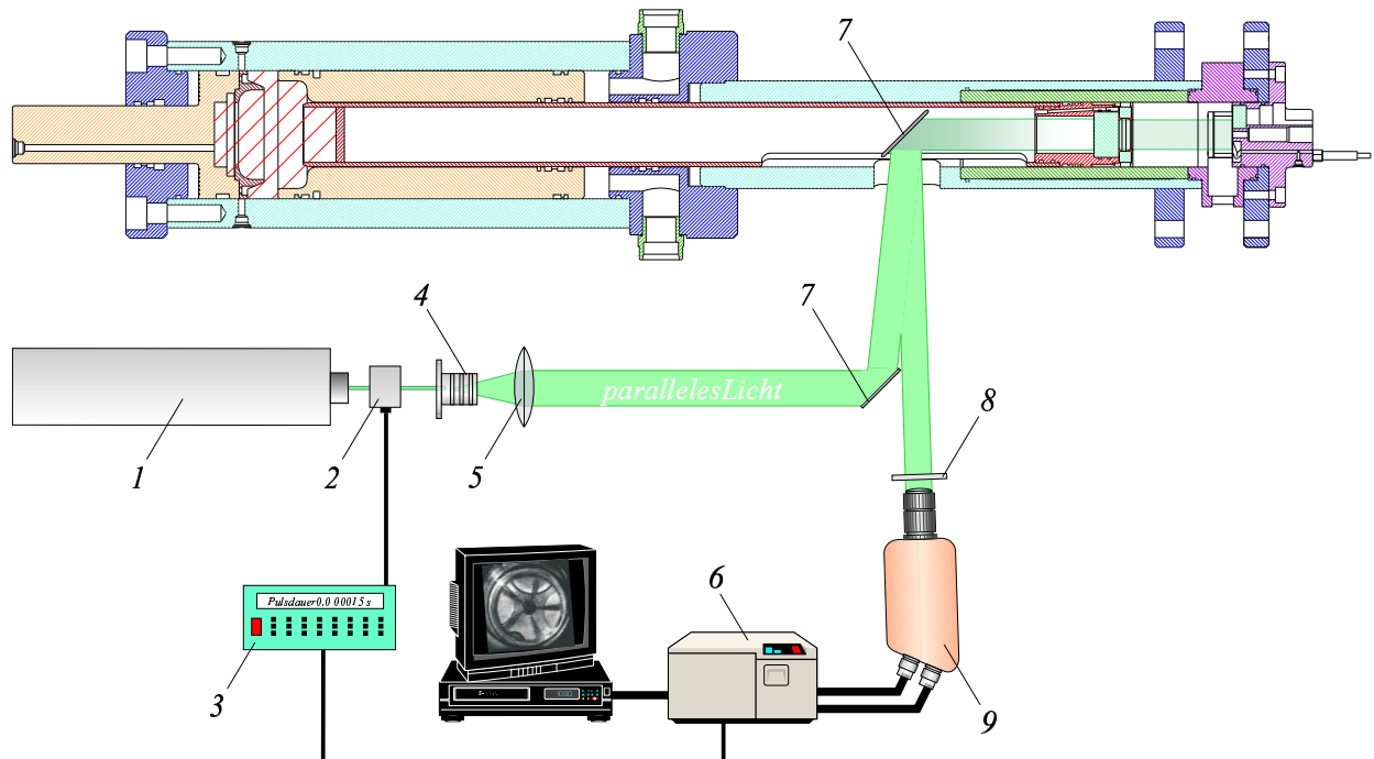
Abbildung 5.3: Verbesserter Meßaufbau der Schattenriß-Kinematographie mit leichter Schrägstellung des Lichtweges
