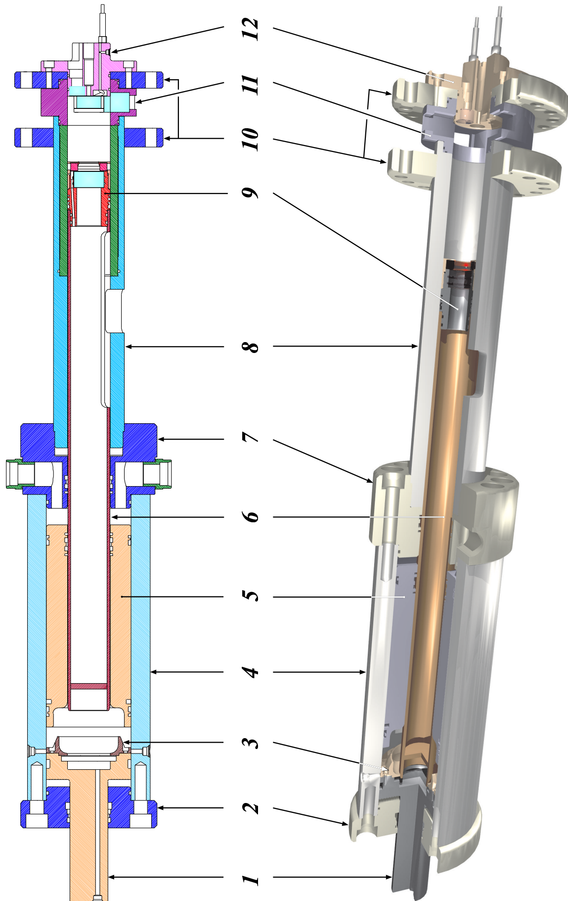
Abbildung D.0: Bauteilübersicht des Einhub-Triebwerks
