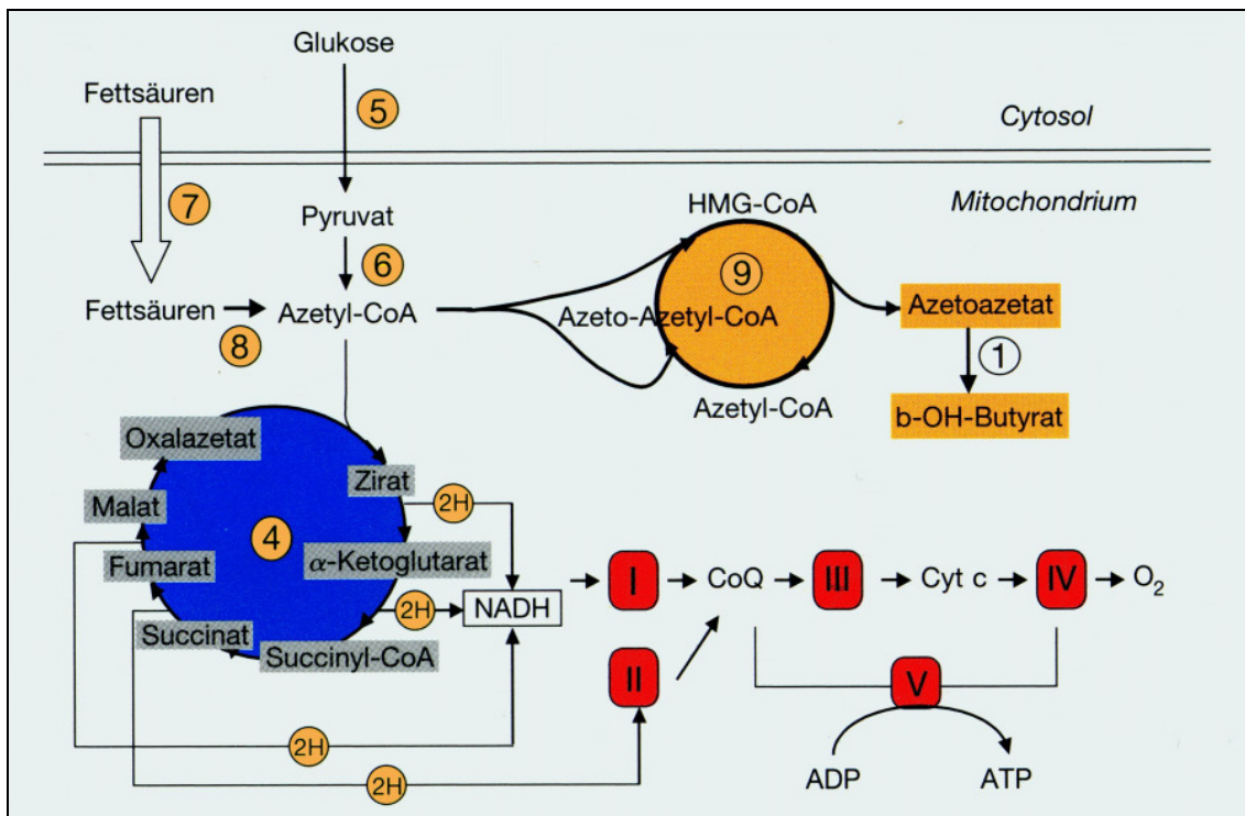
Abbildung 2: Ketogenese
