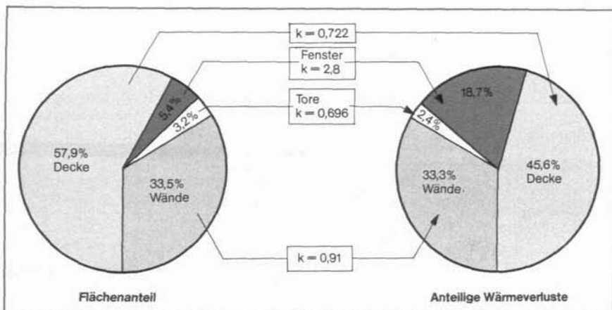
Abb. 79 Einfluß des Wärmedurchgangskoeffizienten verschiedener Stallbauteile auf deren anteilige Wärmeverluste
