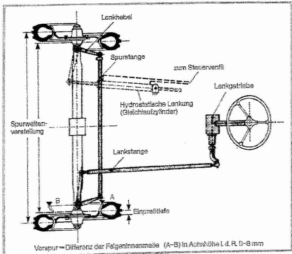
Abb. 55 Aufbau und Funktion einer Achsschenkellenkung
