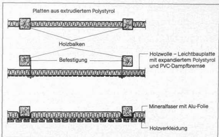
Abb. 100 Aufbau verschiedener Holzbalckendecken
