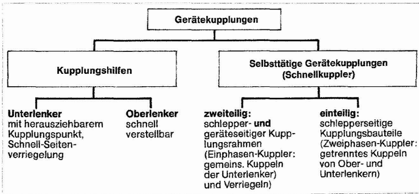
Abb. 63 Übersicht über Gerätekupplungen
