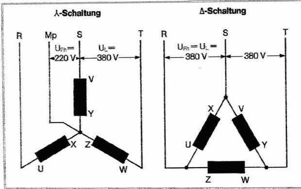
Abb. 13 Schaltarten von Drehstromerzeugern und -verbrauchern (R, S, T = Außenleiter bzw. Phasenleiter, M p = Mittelpunktleiter, U Ph = Phasenspannung, U L = Leiterspannung, U... Z = Wicklungs- bzw. Klemmenbezeichnung)
