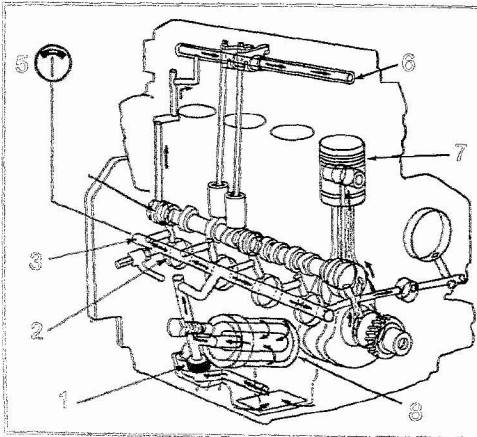
Abb. 31 Schematischer Aufbau einer Schmierung (Druckumlaufschmierung) 1 = Ölpumpe mit Druckregelventil 2 = Kurbelwellenlager 3 = Hauptöl-Verteilerkanal 4 = Nockenwellenlager 5 = Ölmanometer (2–5 bar nach der Pumpe) 6 = Kipphebelwelle 7 = Pleuellagerbuchse und Pleuellager 8 = Ölfilter
