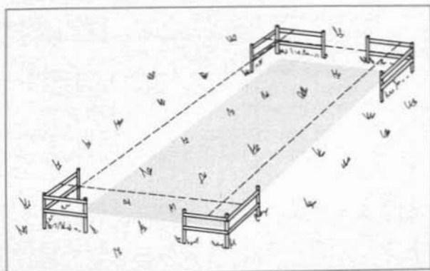
Abb. 136 Einrichtung eines Schnurgerüsts
