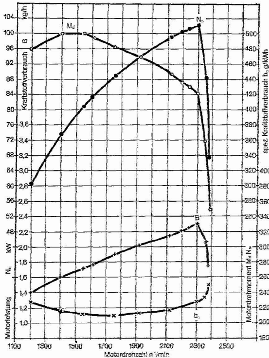
Abb. 32 Vollastkennlinie eines Dieselmotors
