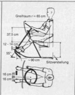
Abb. 148 Richtiger Schlepper-Führerstand
