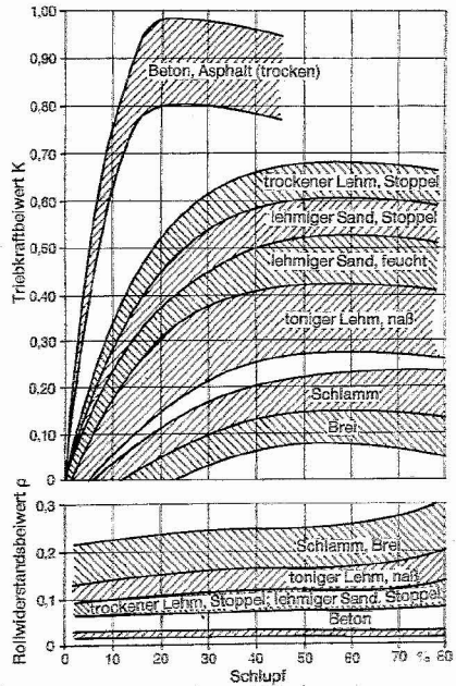
Abb. 52 Triebkraftbeiwerte (oben) und Rollwiderstandsbeiwerte (unten) in Abhängigkeit von Schlupf und Fahrbahn
