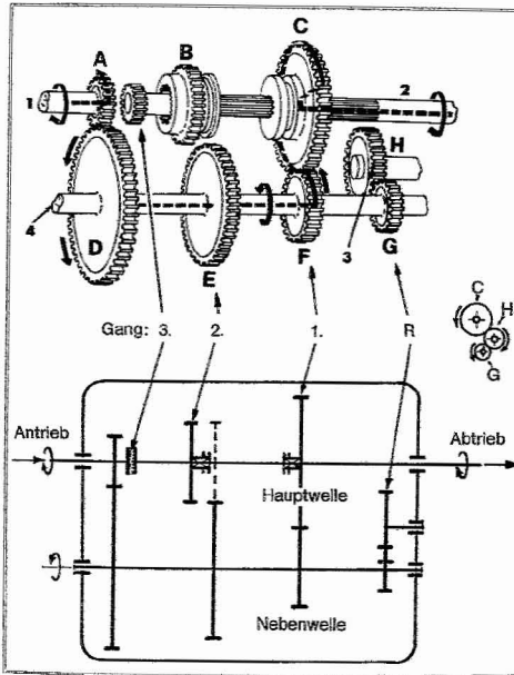
Abb. 41 Aufbau und vereinfachte Darstellung eines Stufengetriebes
