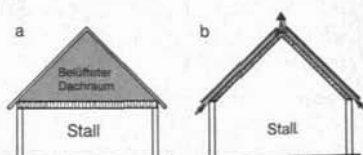
Abb. 99 Kaldtatch; a) mit ebener Decke, b) mit schräger Decke
