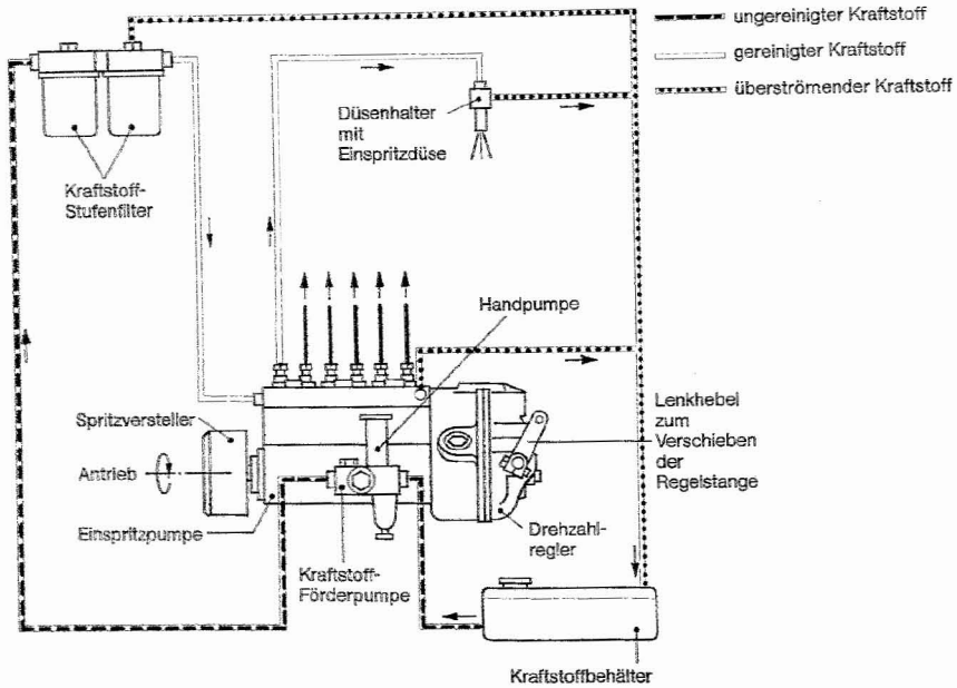
Abb. 24 Die wesentlichen Bestandteile einer Diesel-Einspritzanlage
