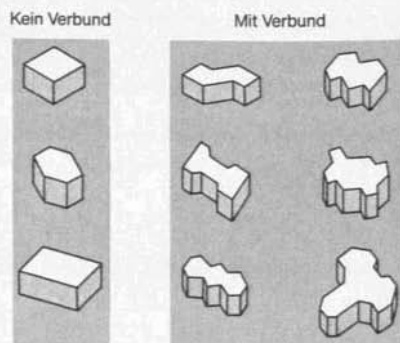
Abb. 87 Beispiele für Betonpflastersteine
