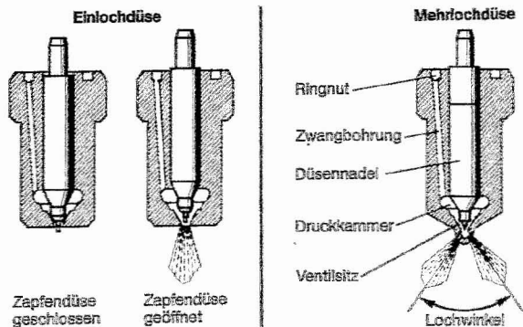
Abb. 27 Aufbau und Wirkung einer Einloch- und Mehrlochdüse
