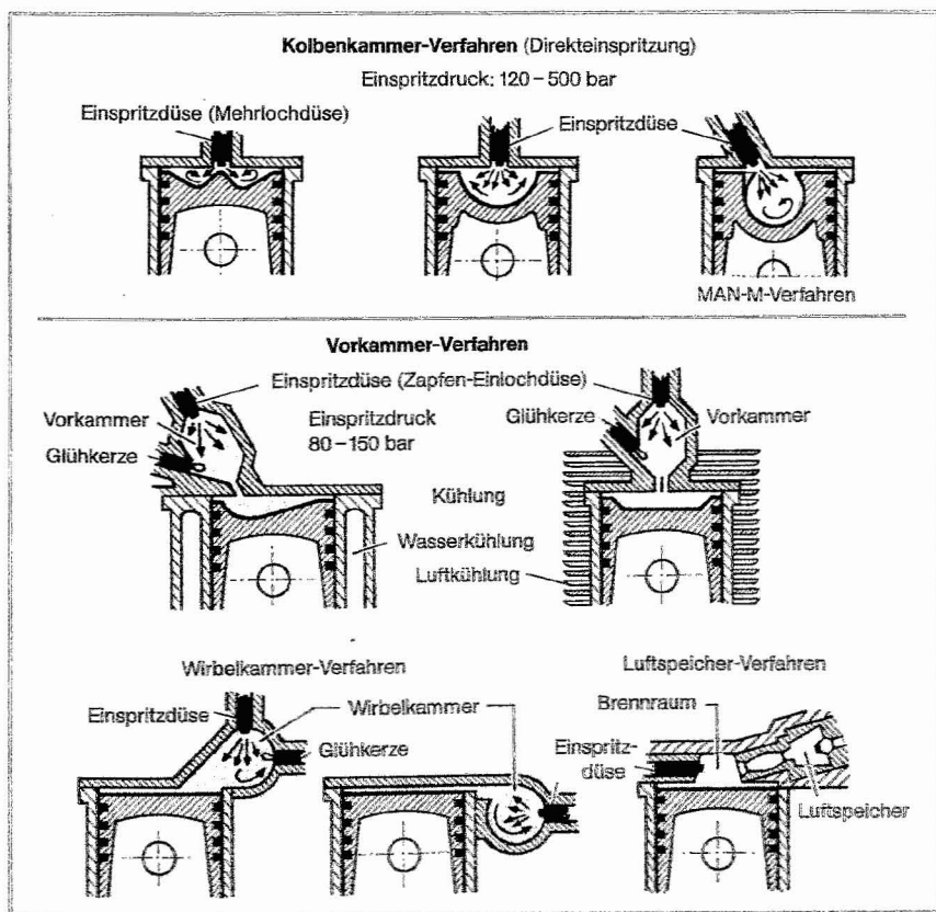
Abb. 22 Einspritzverfahren beim Dieselmotor
