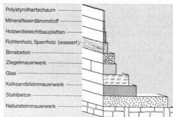
Abb. 82 Materialdicke bei gleicher Wärmedämmung ( k = 0,95 \text{ W/m}^2 \text{ K} )
