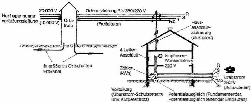
Abb. 18 Schema einer Elektroinstallation
