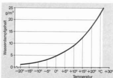
Abb. 83 Maximaler Wasserdampfgehalt der Luft in Abhängigkeit von der Temperatur
