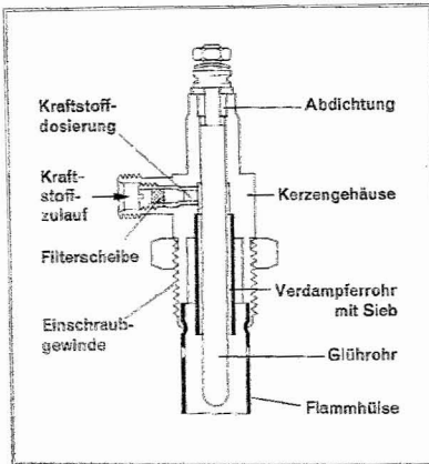
Abb. 28 Aufbau einer Flammglühkerze
