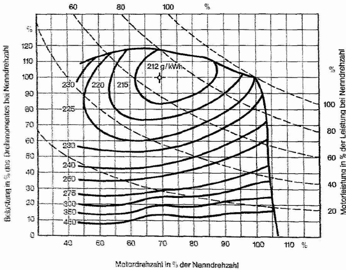
Abb. 33 Motorkennfeld eines Dieselmotors
