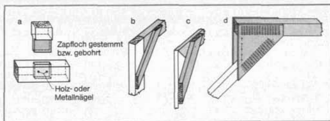
Abb. 92 Holzverbindungen:
