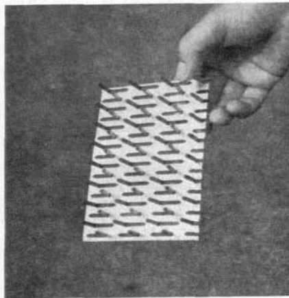
Abb. 94 Verzinkte Holzverbinder: Nagelplatte (Gang-Nail-Platte)
