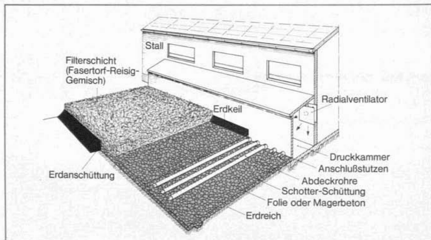
Abb. 124 Erdfilteranlage
