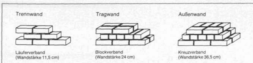
Abb. 88 Mauerverbände (Normalsteine) unterschiedlicher Funktion
