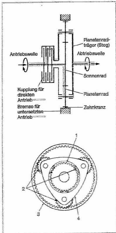
Abb. 46 Aufbau und Funktion eines Lastschalt-Vierganggetriebes mit Planetensatz 1 = Sonnenrad 2 = Planetenrad 3 = Hohlrad (Zahnkranz) 4 = Planetenradträger (Steg)
