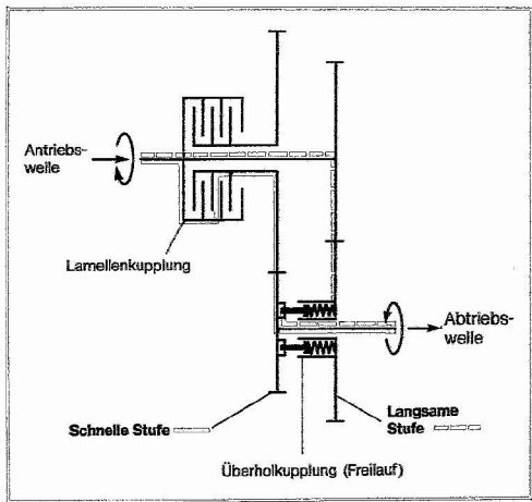
Abb. 45 Aufbau und Funktion eines Lastschaltgetriebes mit Überholkupplung
