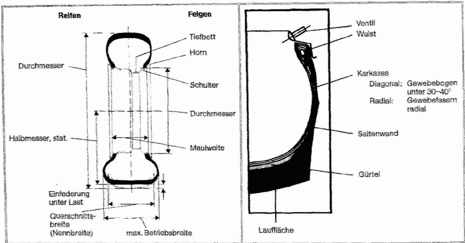
Abb. 54 Grundsätzlicher Aufbau eines Reifens und einer Felge
