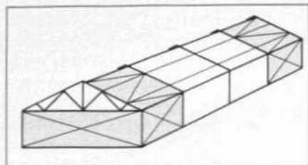
Abb. 105 Windverband eines Gebäudes
