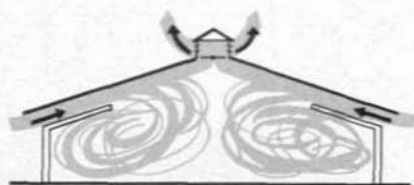
Abb. 118 Trauf-First-Lüftung
