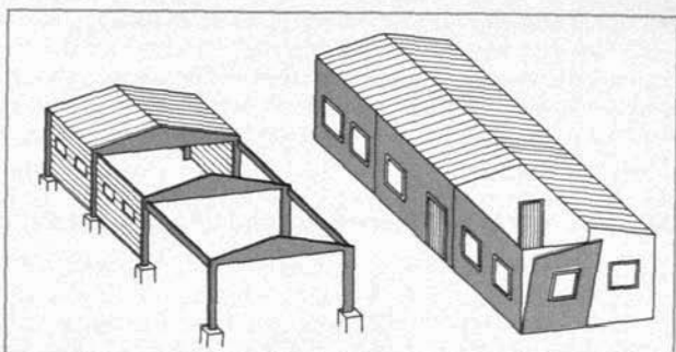
Abb. 107 (l) Skelettbauweise, (r) Mantelbauweise
