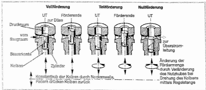
Abb. 25 Wirkungsweise einer Reiheneinspritzpumpe
