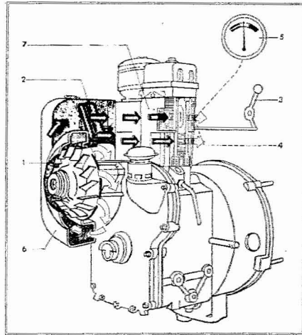
Abb. 29 Schema einer Luftkühlung 1 Gebläsead, 2 Drosselklappe, 3 Handhebel zur Drosselklappenverstellung, 4 Temperaturegeber für Thermometer, 5 Thermometer (am Armaturenbrett), 6 Kühlluftgebläse, 7 Luftleitbleche
