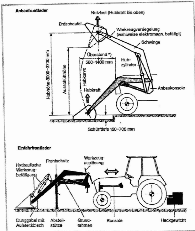
Abb. 65 Grundsätzlicher Aufbau eines Schlepper-Frontladers
