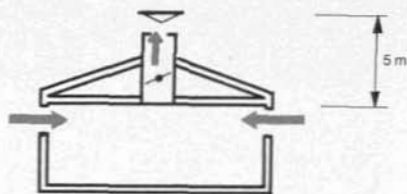
Abb. 117 Schachtlüftung
