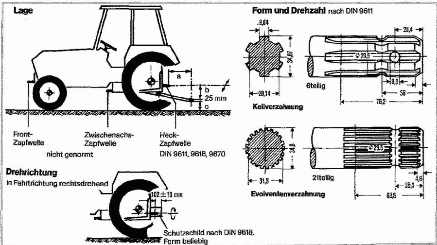
Abb. 66 Genormte Teile an der Schlepperzapfwelle
