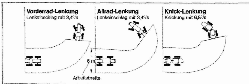
Abb. 56 Schlepperkurven bei verschiedenen Lenkungsarten
