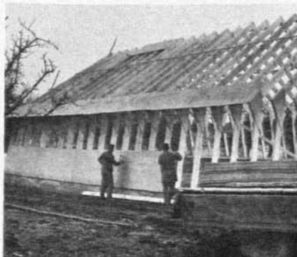
Abb. 110 Starrahmenbauweise
