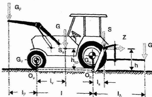
Abb. 37 Kräfte am Schlepper
