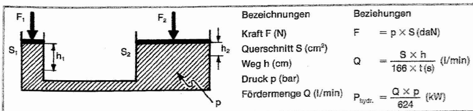
Abb. 60 Grundlagen der Hydrostatik
