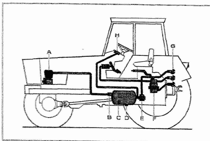
Abb. 57 Aufbau einer Druckluftfüllanlage
