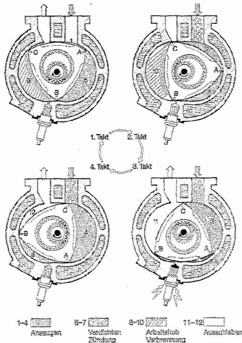
Abb. 21 Arbeitspiel eines Kreiskolbenmotors
