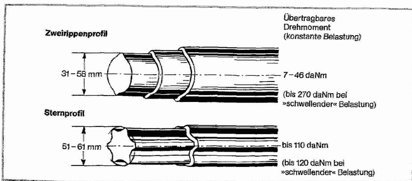
Abb. 69 Profilierung von Gelenkwellen
