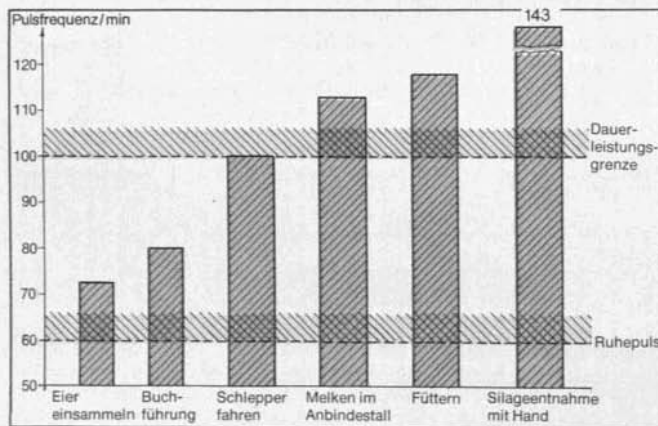
Abb. 144 Belastung bei einigen landwirtschaftlichen Arbeiten
