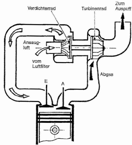
Abb. 23 Funktion eines Abgasturboladers
