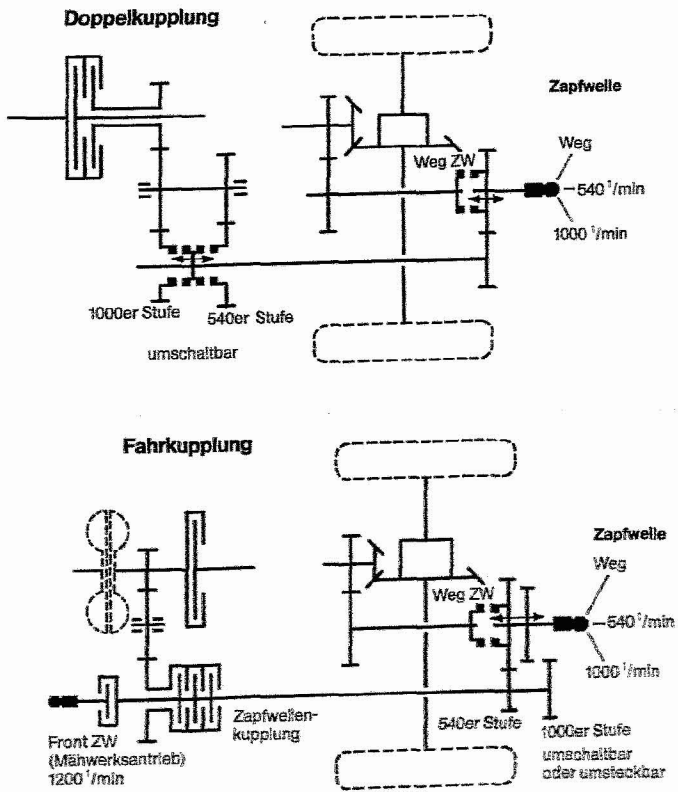
Abb. 66 Genormte Teile an der Schlepperzapfwelle
