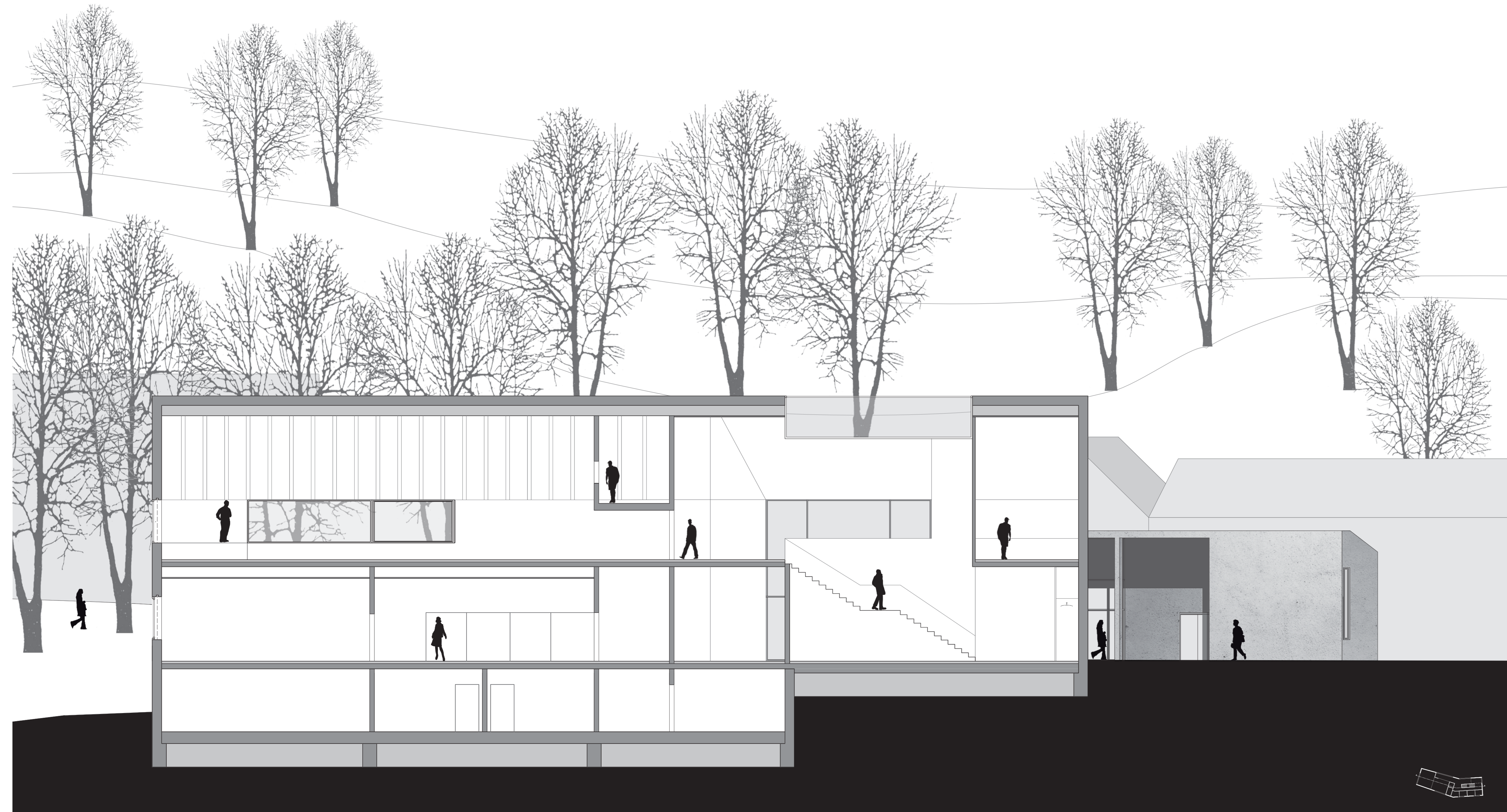
Längsschnitt M 1:100
