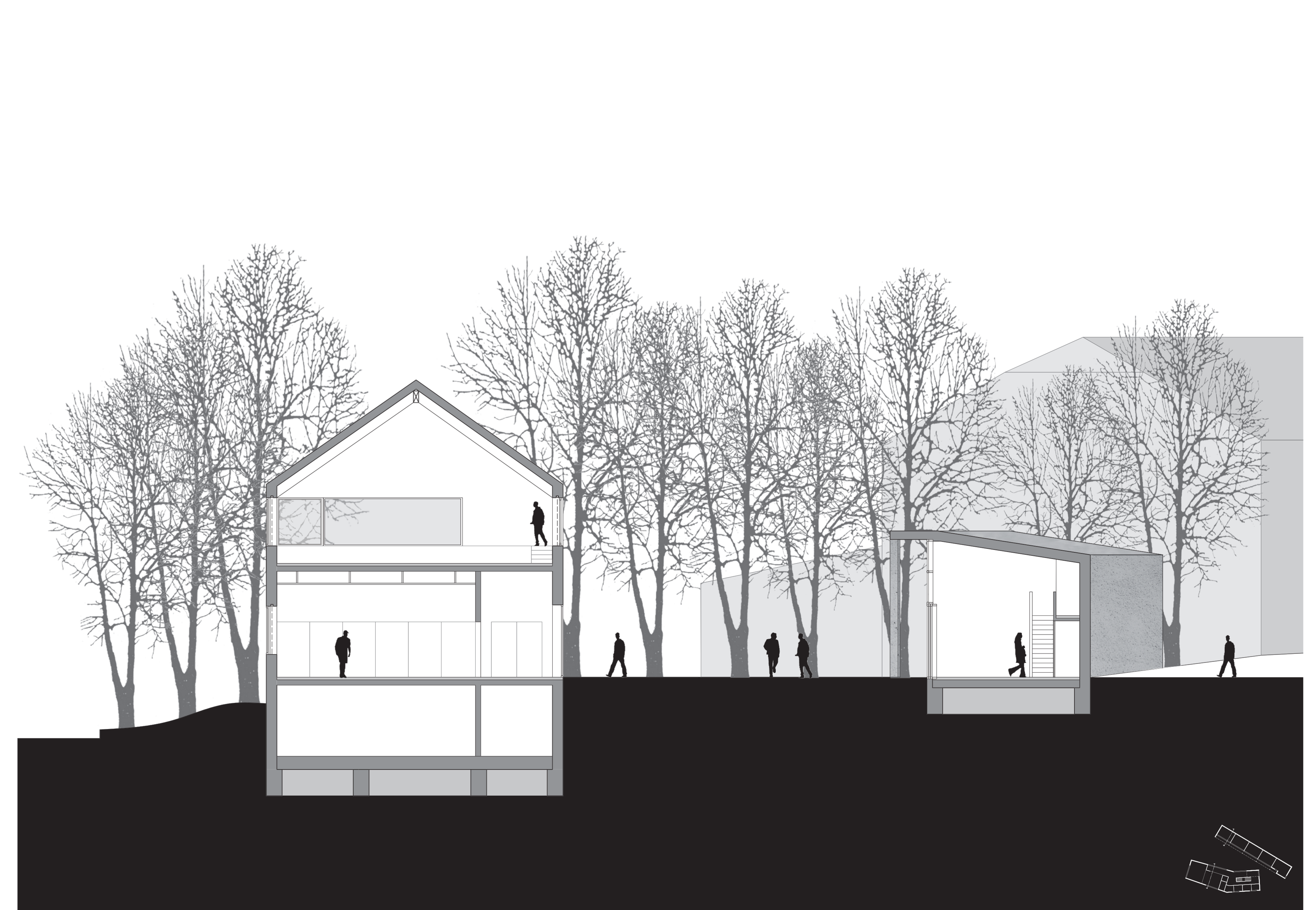
Querschnitt M 1:100
