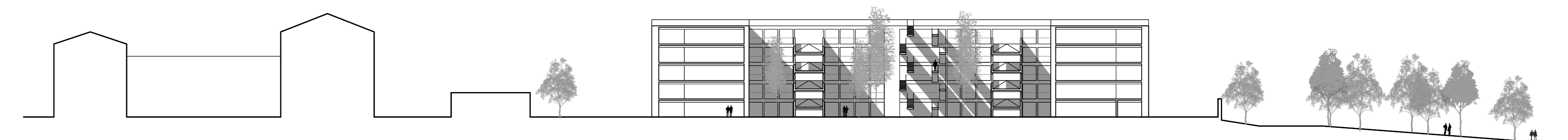
SCHNITT A-A 1/500
