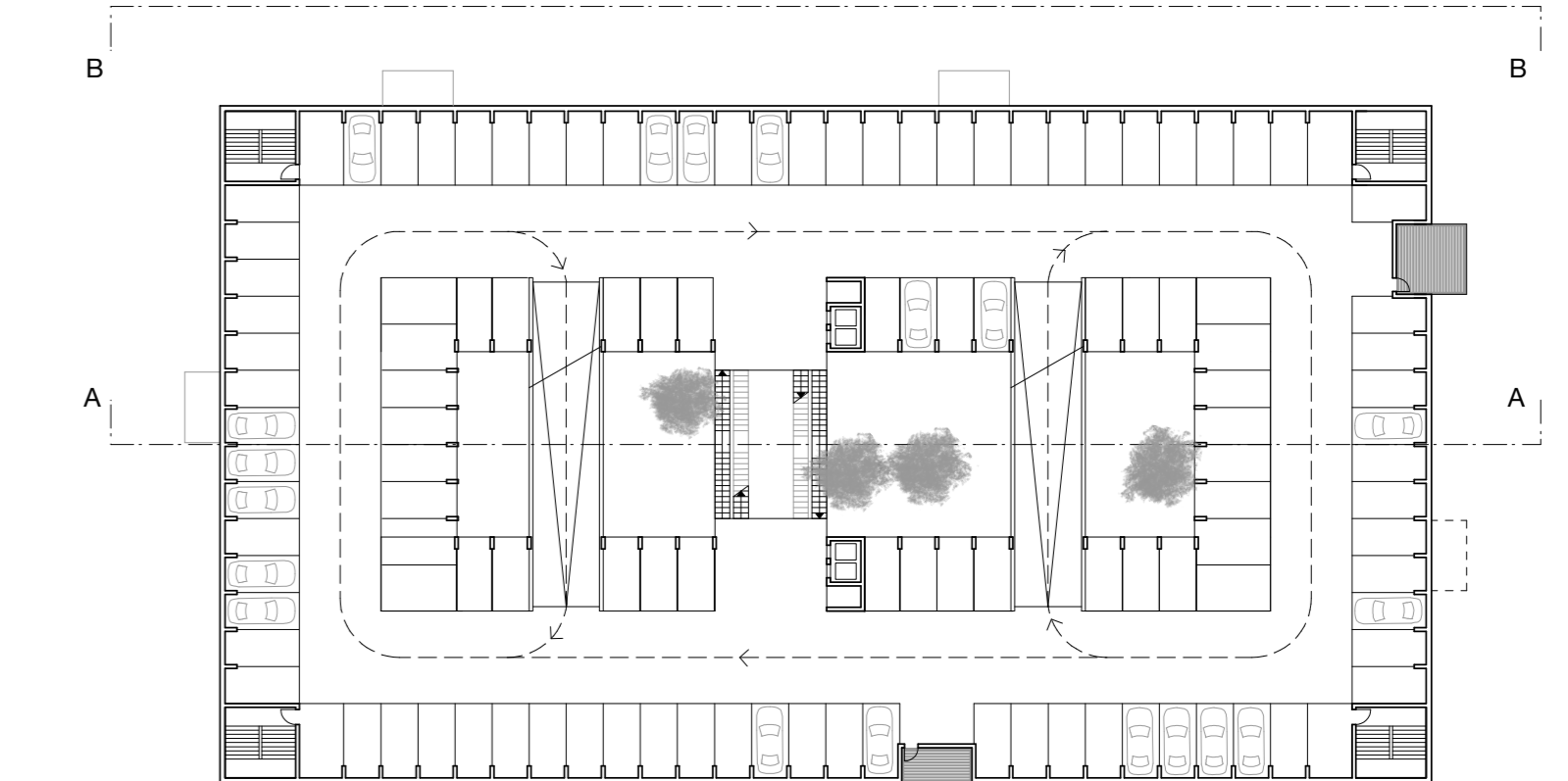
GRUNDRISS REGELGESCHOSS 1/500
