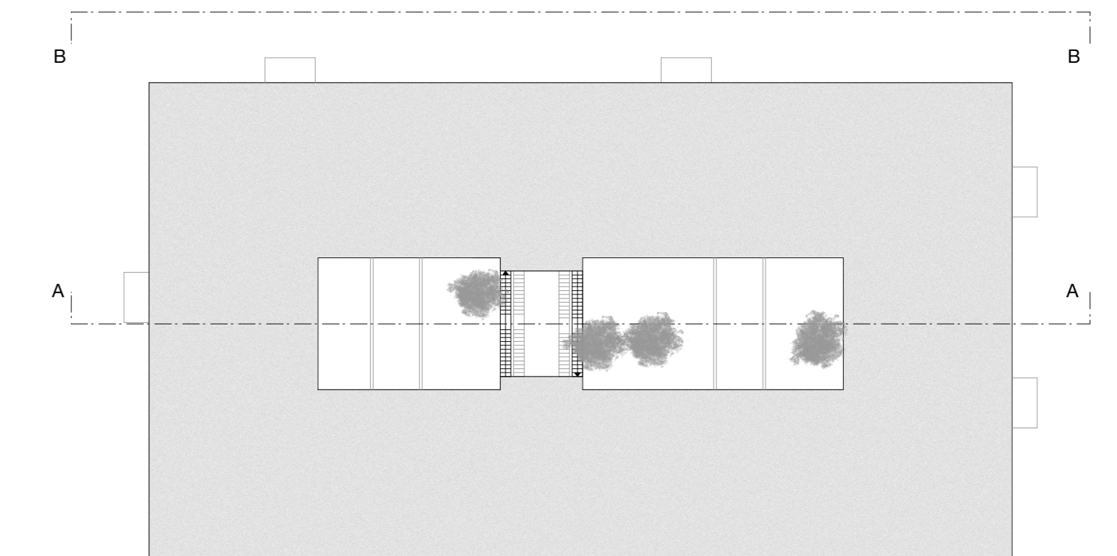
DACHAUFSICHT 1/500
