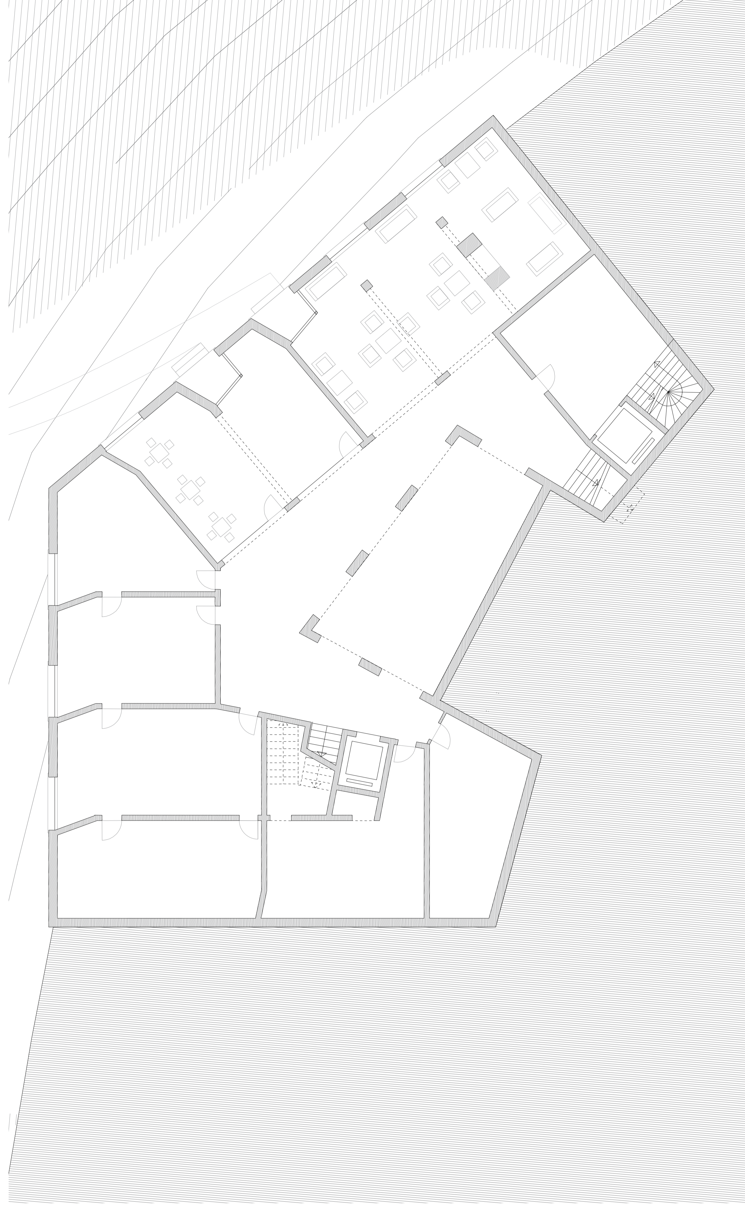
grundriss eg 1_100 verwaltung_kinderbetreuung_untere lobby_kaminzimmer
