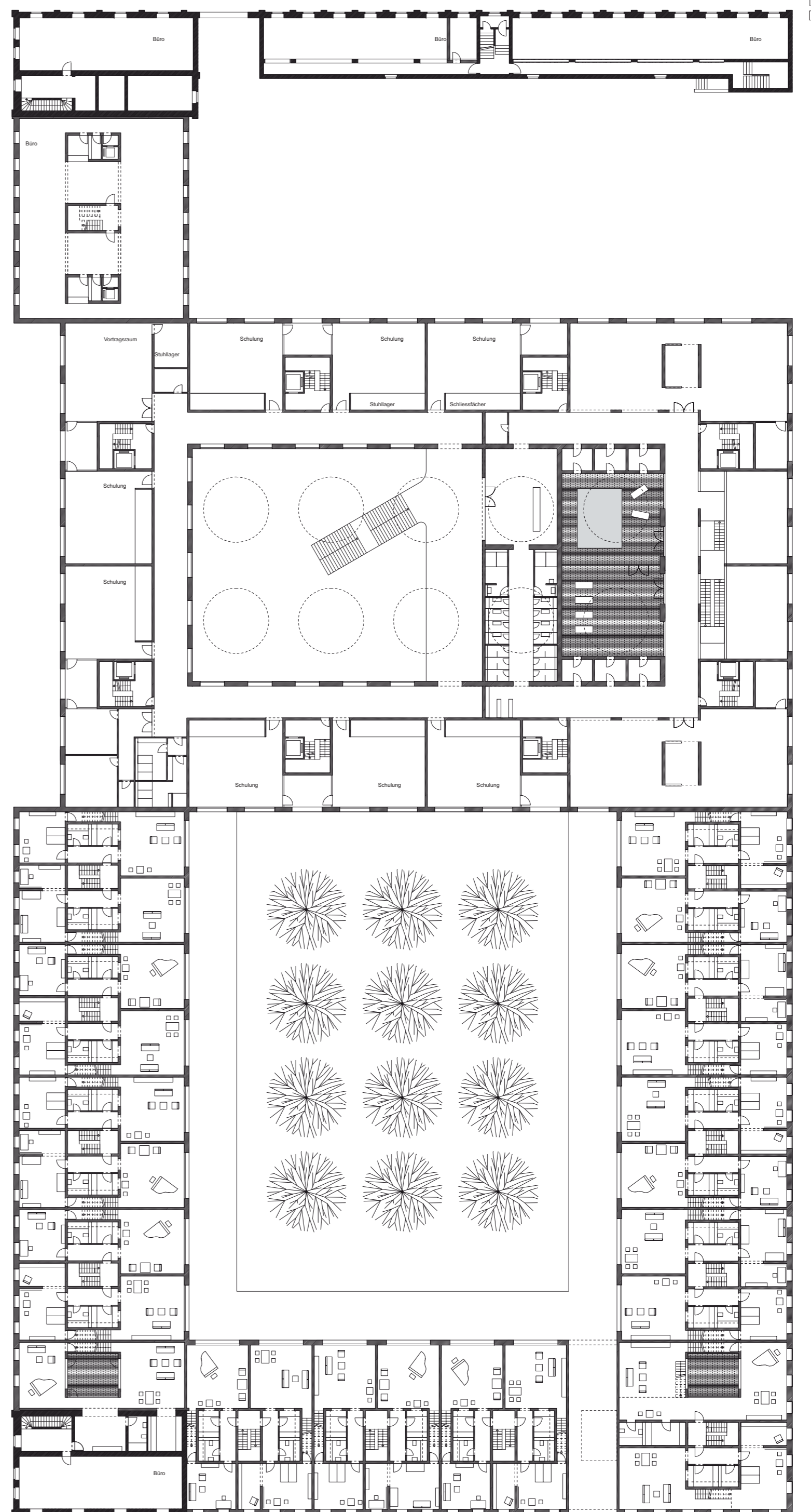
GRUNDRISS 1. OBERGESCHOSS M 1_200
