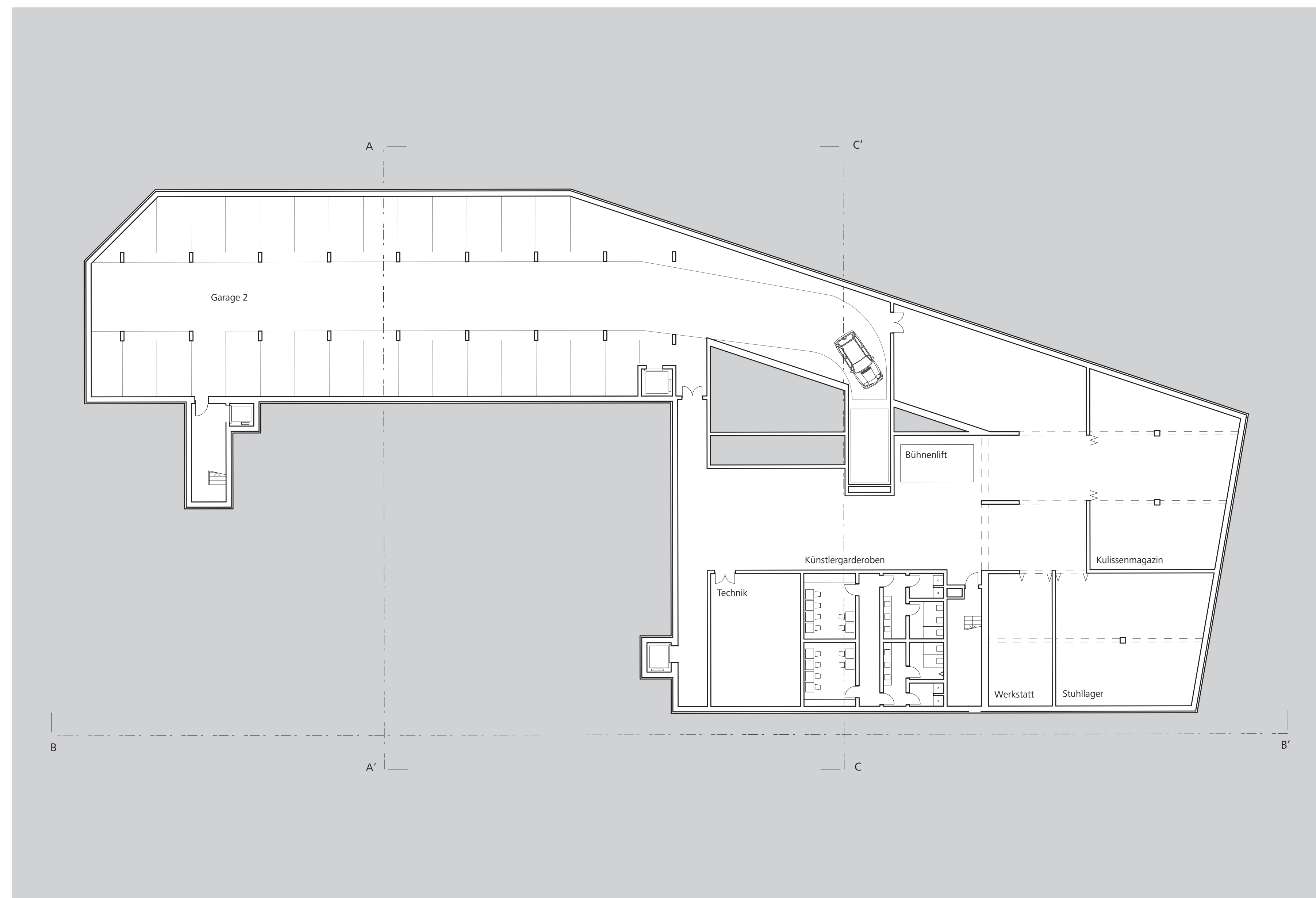
Tiefgeschoss M 1:200
