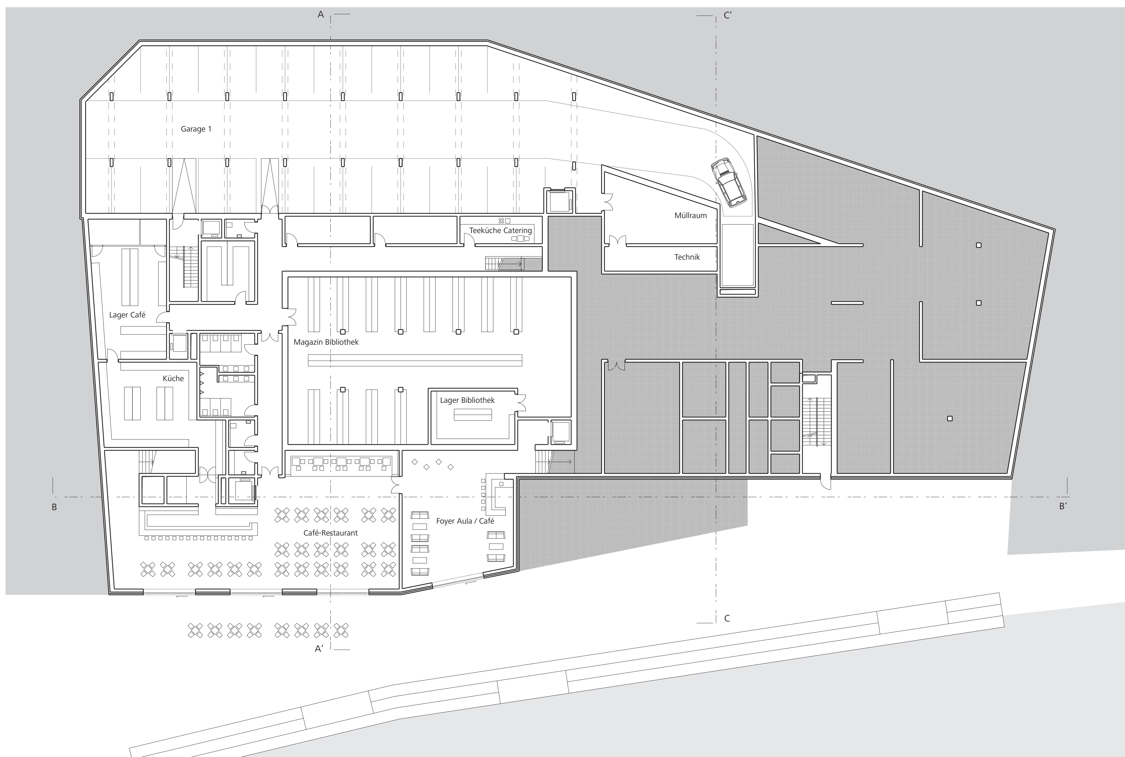
Ufergeschoss M 1:200
