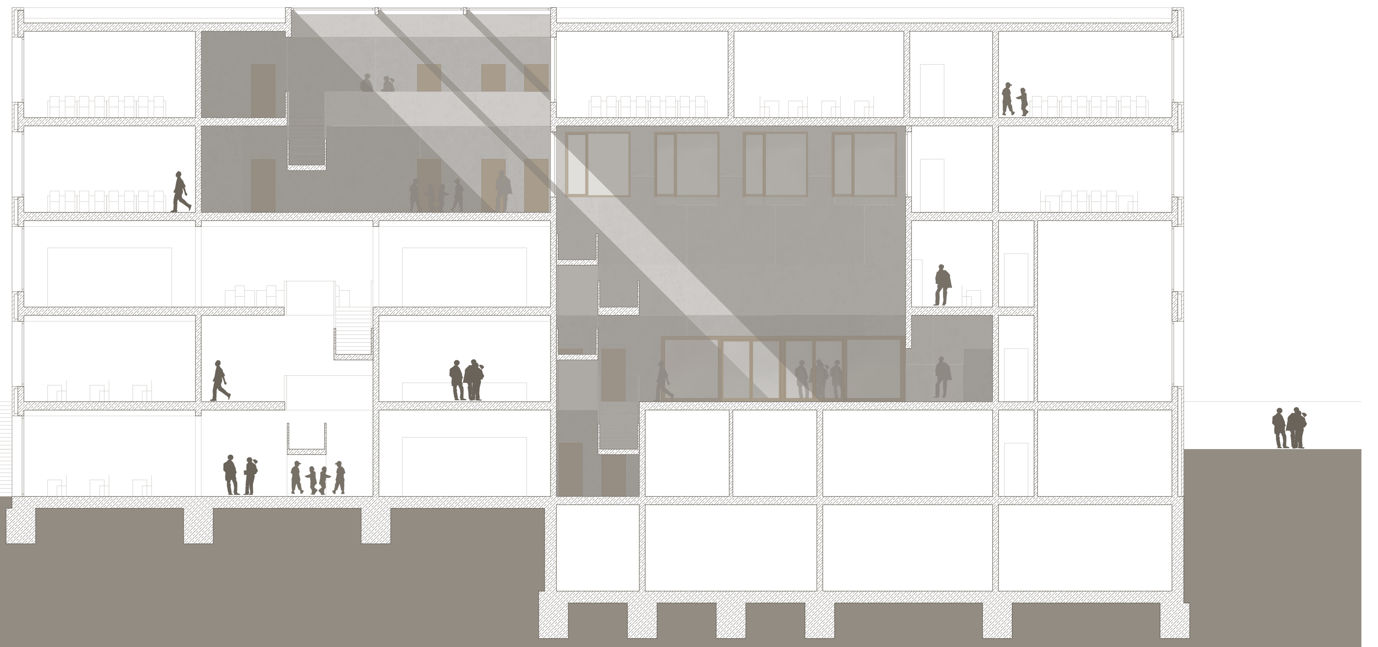
Schnitt A - A M 1:100
