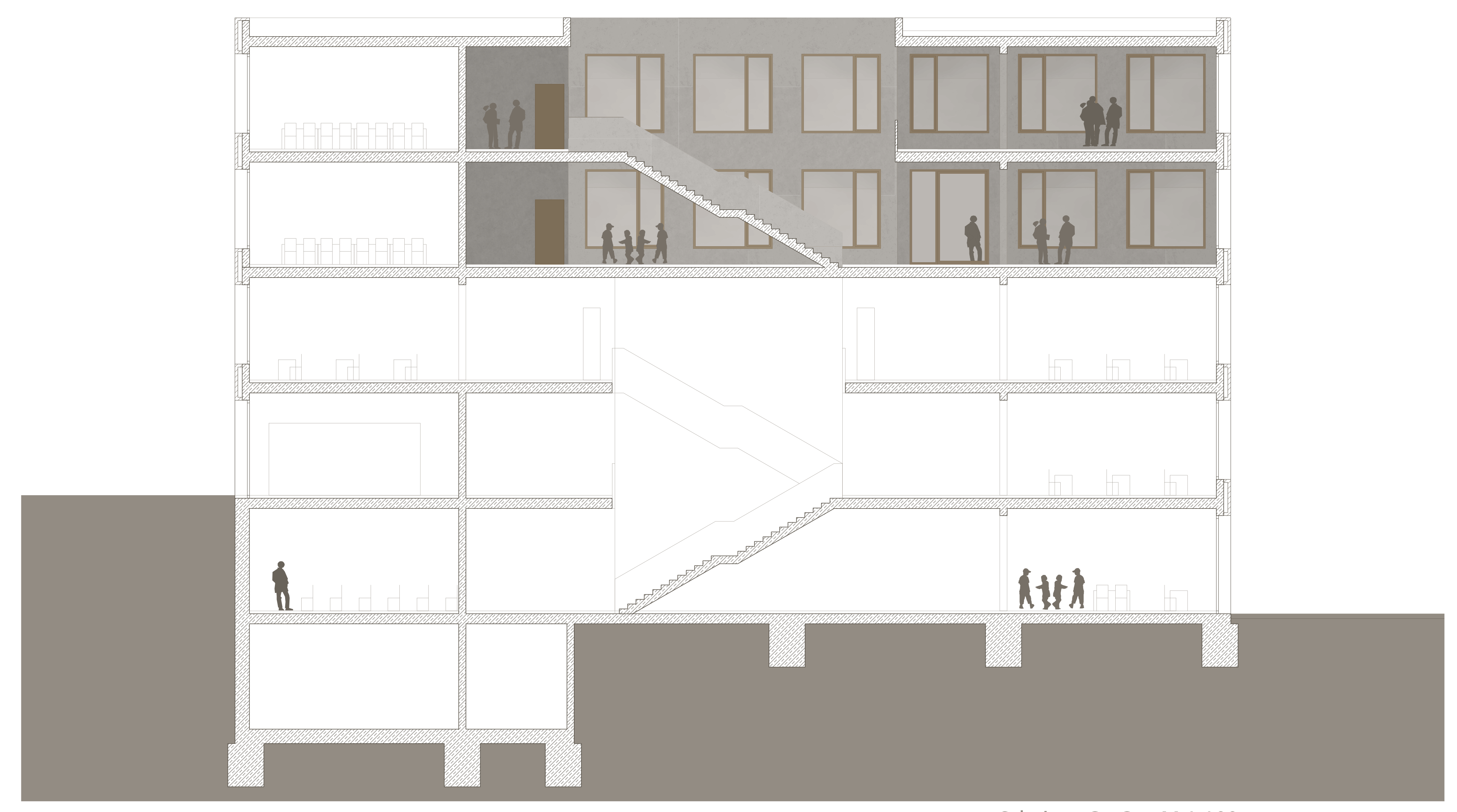
Schnitt C - C M 1:100
