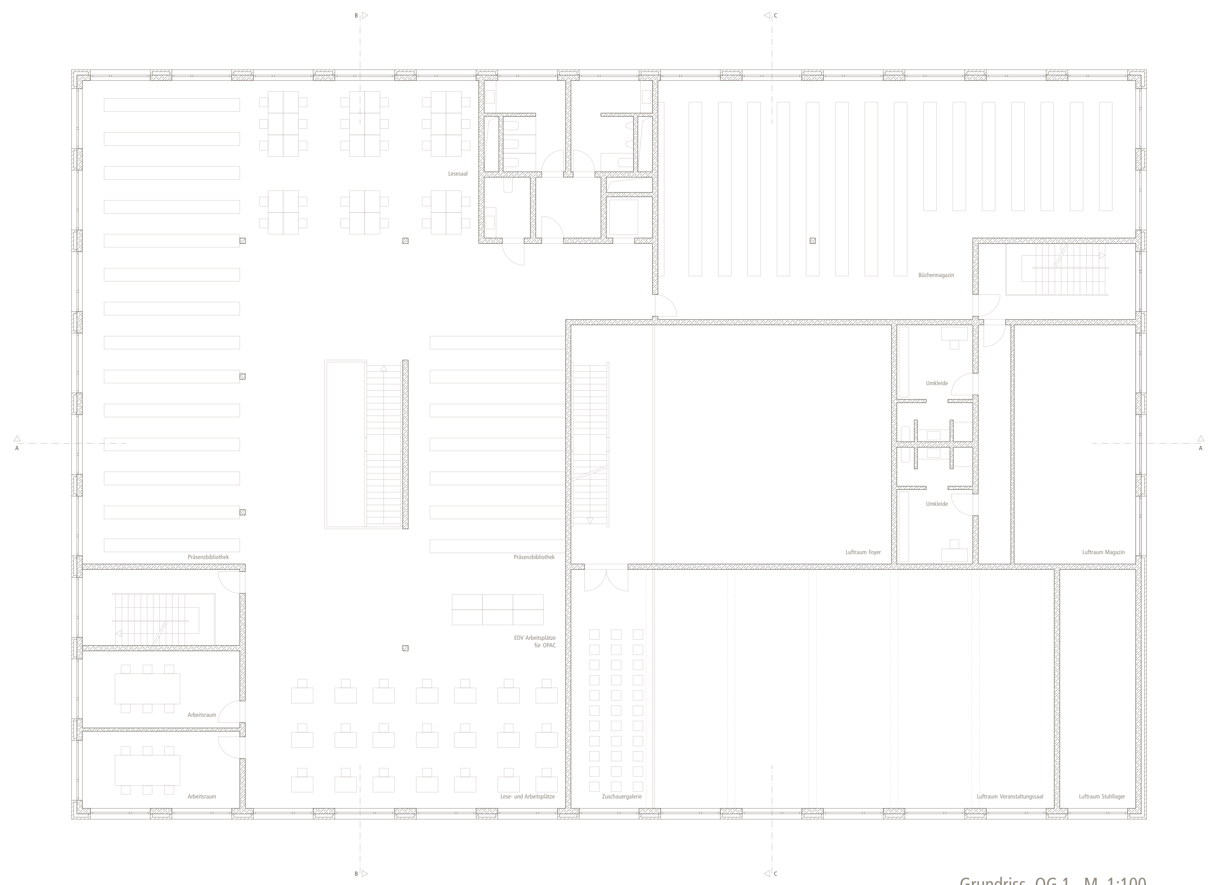
Grundriss OG 1 M 1:100
