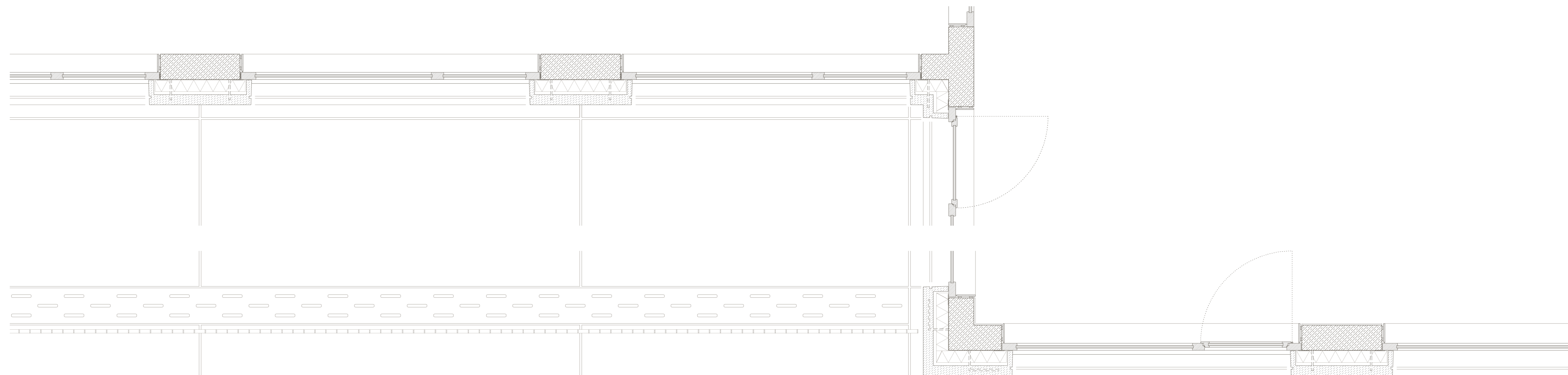
Fassadengrundriss M 1:20
