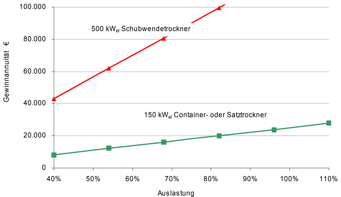
Abbildung 4-2: Gewinnannuität der Hackschnitzel trocknung in Abhängigkeit der Auslastung. Berücksichtigt sind alle Kosten und Einnahmen der Wärmenutzungsvariante und der KWK-Bonus.
