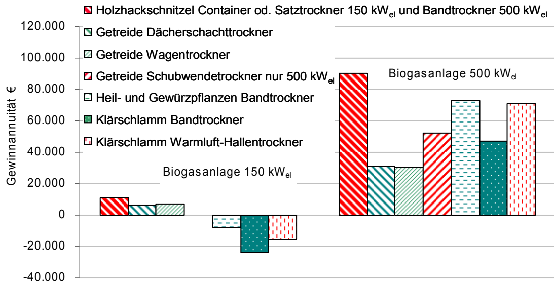
Abbildung 4-1: Gewinnannuität der untersuchten Trocknungsprozesse. Berücksichtigt sind alle Kosten und Einnahmen der Wärmenutzungsvariante und der KWK-Bonus.
