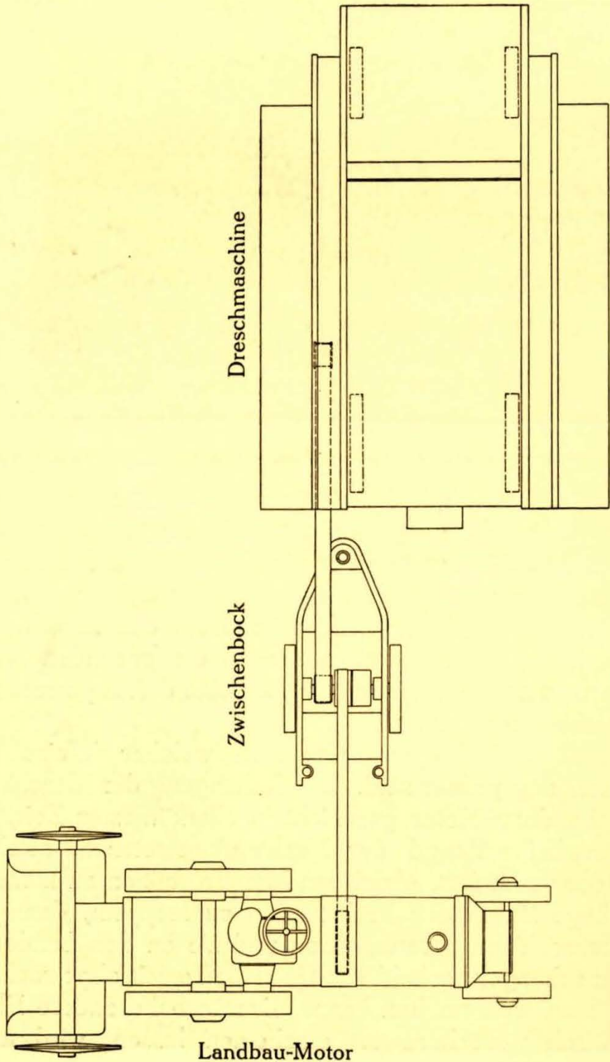
LANDBAU-MOTOR LANZ TREIBT EINEN DRESCHSATZ
