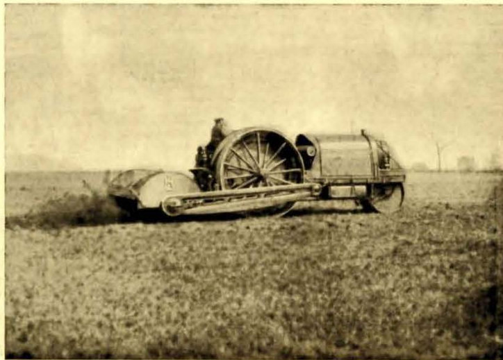
LANDBAU-MOTOR LANZ, SYSTEM KÖSZEGI. — BAUART 1912/13.
