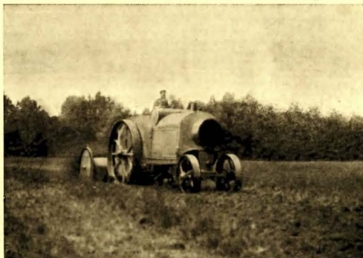
LANDBAU-MOTOR LANZ, SYSTEM KÖSZEGI. — BAUART 1914.
