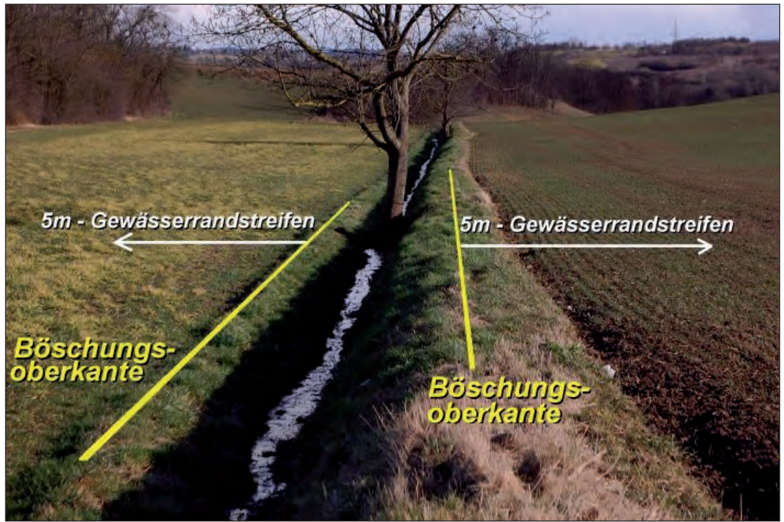
Feststellung des 5 m Bereiches zur Böschungsoberkante
