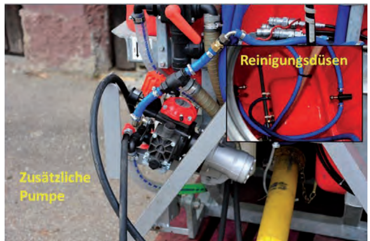
Kontinuierliche Innenreinigung
