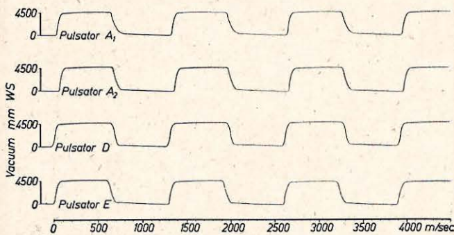
Abb. 6: Beispiele von Pulscurven verschiedener Pulsatoren, aufgenommen mit der Registrierkamera
