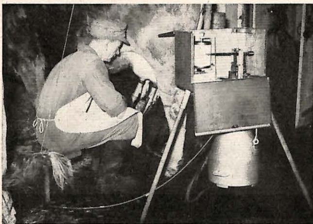
Abb. 7: Der Melkleistungsschreiber im Einsatz
