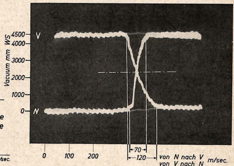
Abb. 2: Oszillogramm der Pulskurve eines Pulsators mit hoher Melkgeschwindigkeit
