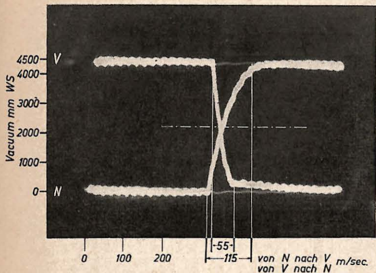
Abb. 3: Oszillogramm der Pulskurve eines Pulsators mit niedriger Melkgeschwindigkeit
