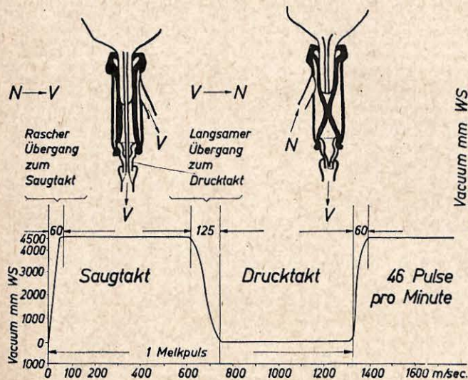
Abb. 1: Darstellung einer Pulskurve
