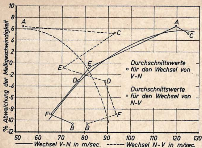
Abb. 12: Bewertungskurve für Pulsatoren
