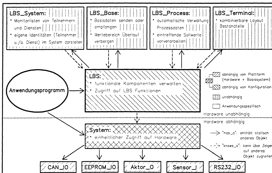
Abbildung 1: Darstellung der LBS Lib im Vollausbau
