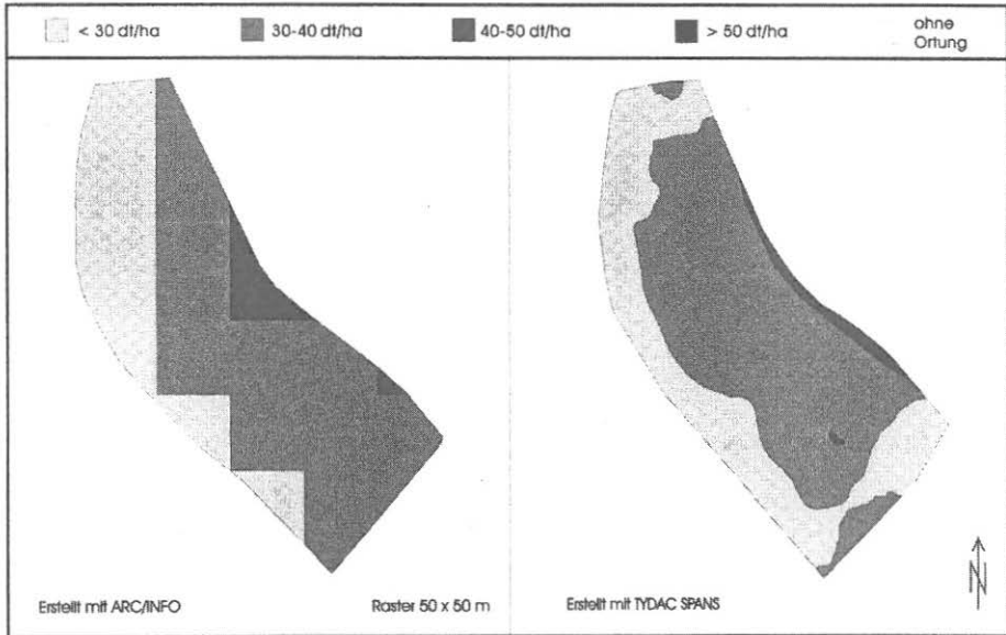
Abbildung 6: Ertragskartierung nach Rasterflächen bzw. Isoertragsflächen Scheyern Eulenwies 1992 (S-Gerste, mittlerer Ertrag 34 dt/ha, Ertragsermittlung DATAVISION FLOWCONTROL, Ortung ASH-TECH / TRIMBLE DGPS).
