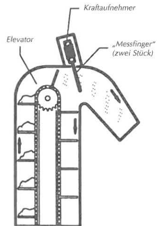
Abbildung 5: Arbeitsweise des FIELDSTAR N-SET Ertragsmessgerätes von AGCO / DRONNINGBORG .
