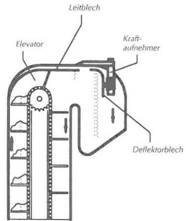
Abbildung 3: Arbeitsweise des YIELD MONITOR YM2000/PF3000 Ertragsmessgerätes von AGLEADER (baugleich LH 565/LH665 von LH AGRO bzw. Sensoranordnung identisch AFS von CASE und TCS von DEUTZ FAHR ).
