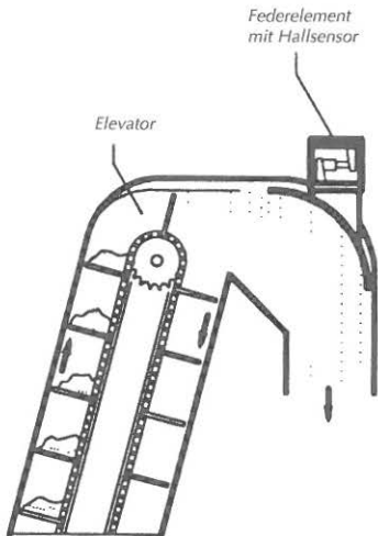
Abbildung 4: Arbeitsweise des GREENSTAR Ertragsmessgerätes von JOHN DEERE .
