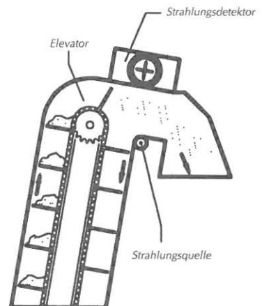
Abbildung 2: Arbeitsweise des DATAVISION-FLOWCONTROL / FIELDSTAR Ertragsmessgerätes von MASSEY FERGUSON / FENDT .
