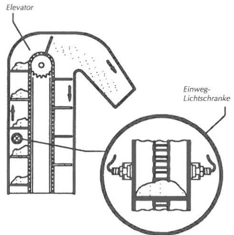
Abbildung 1: Arbeitsweise des QUANTIMETER Ertragsmesssystems von CLASS bzw. CERES 2 /PRO SERIES 8000 Ertragsmessgerätes von RDS.
