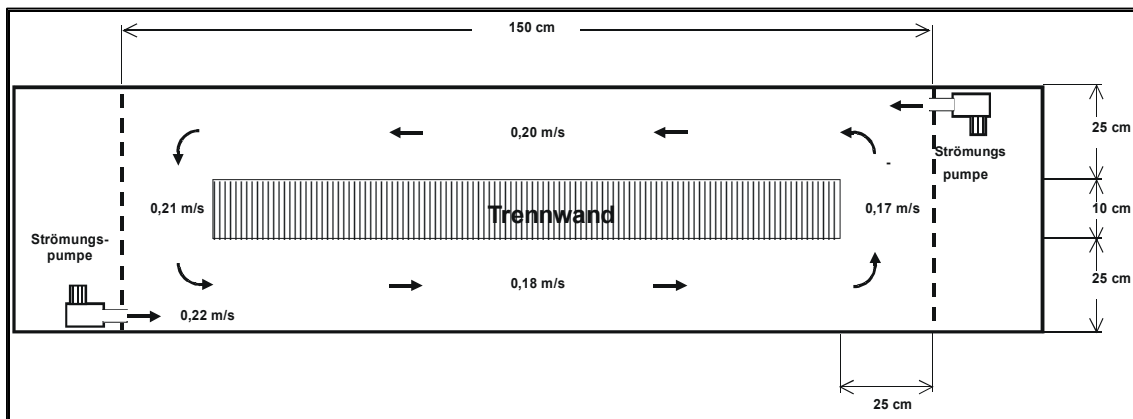
Abb. 45: Strömungsbecken schematisch (SCHUBERT 2001 2 )
