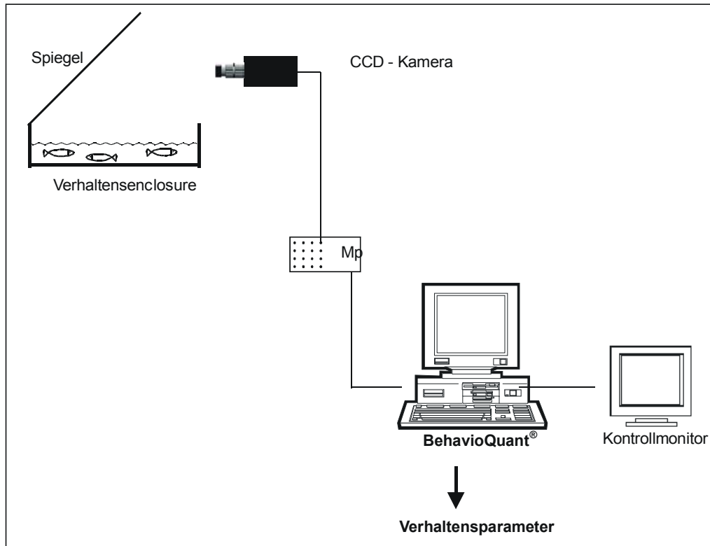
Abb. 46: Schematische Darstellung des Messsystems BehavioQuant® (SCHUBERT 2001 2 )
